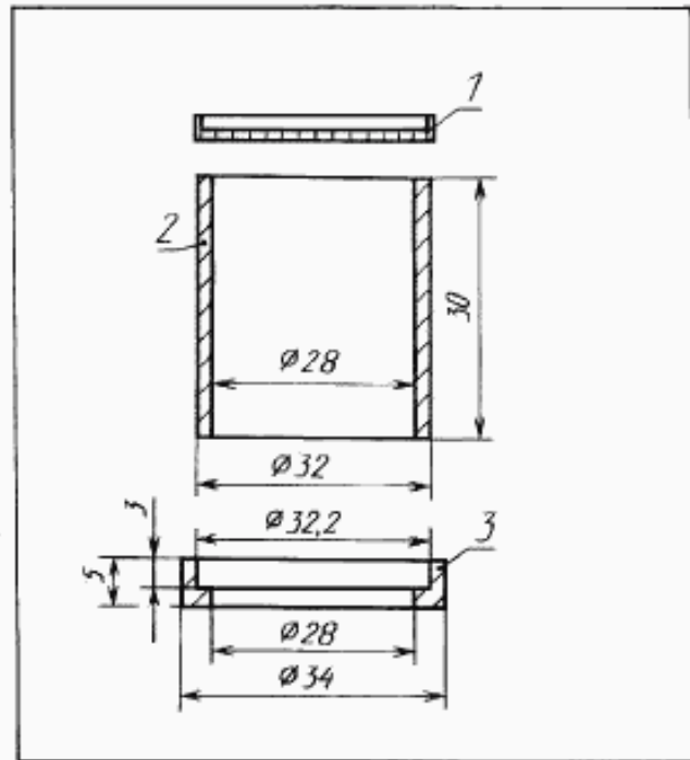
Фильтрующее устройство
