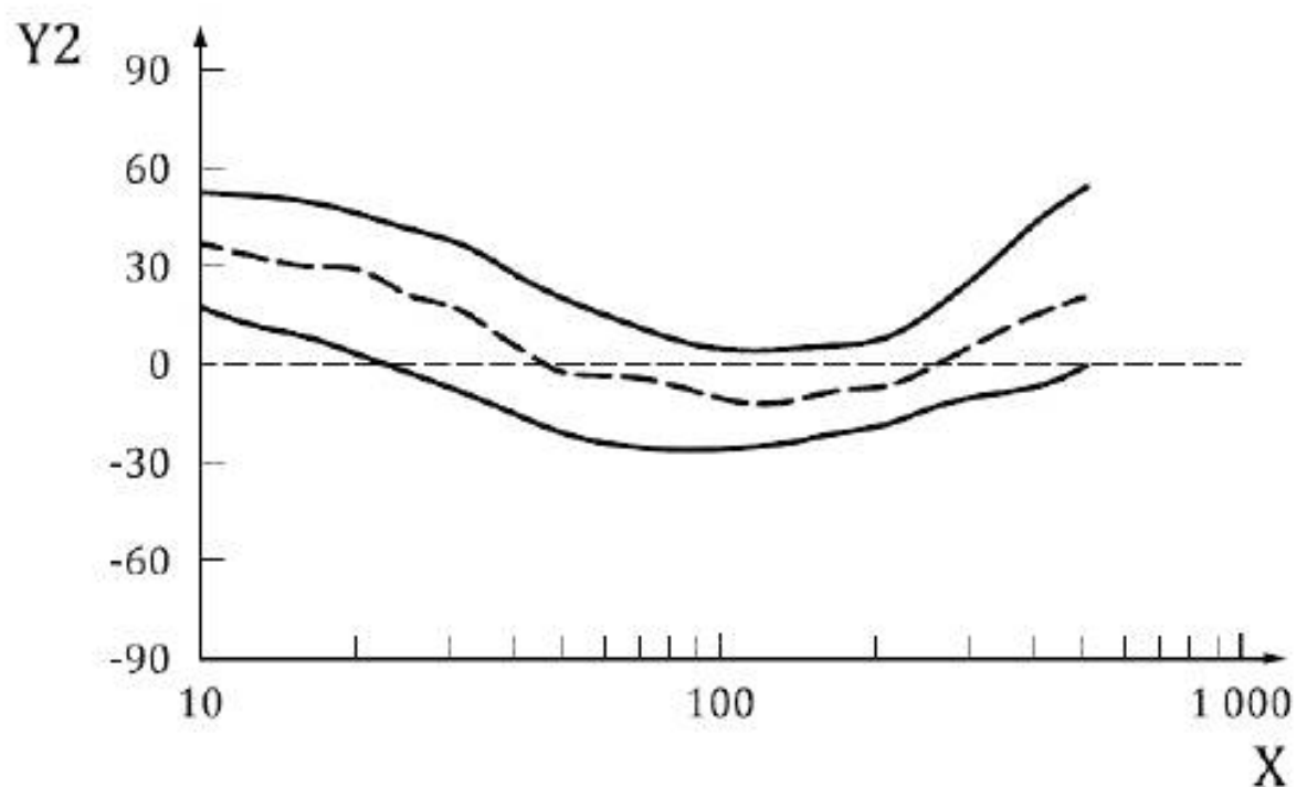
Рисунок 2 — Значения входного механического импеданса для системы «кисть — рука» в направлении y_0
