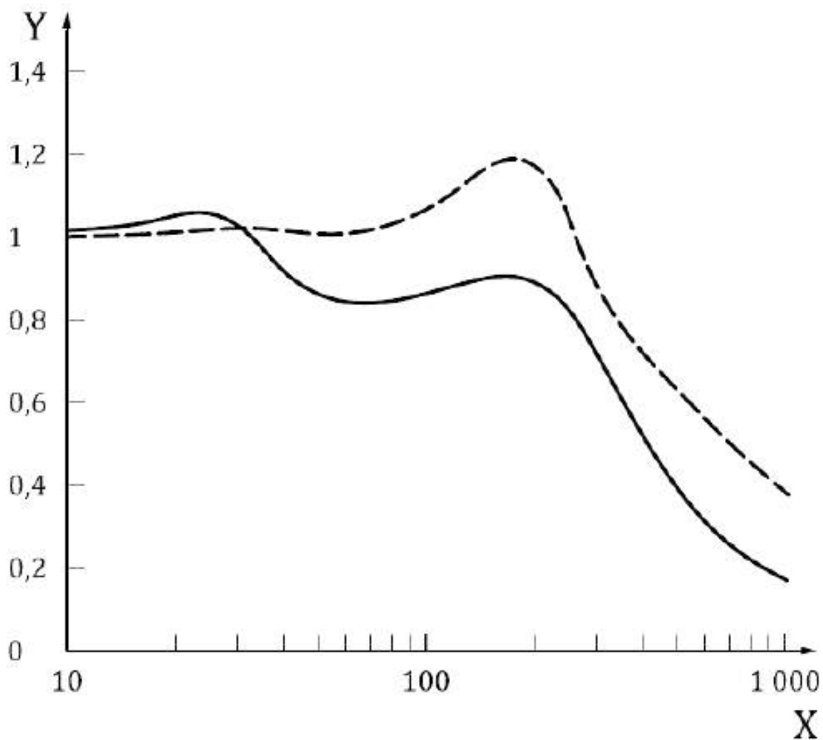
Рисунок Е.2 — Предсказанный моделью коэффициент передачи перчаток в области пальцев (сплошная линия) и ладони (пунктирная линия) в направлении z_1
