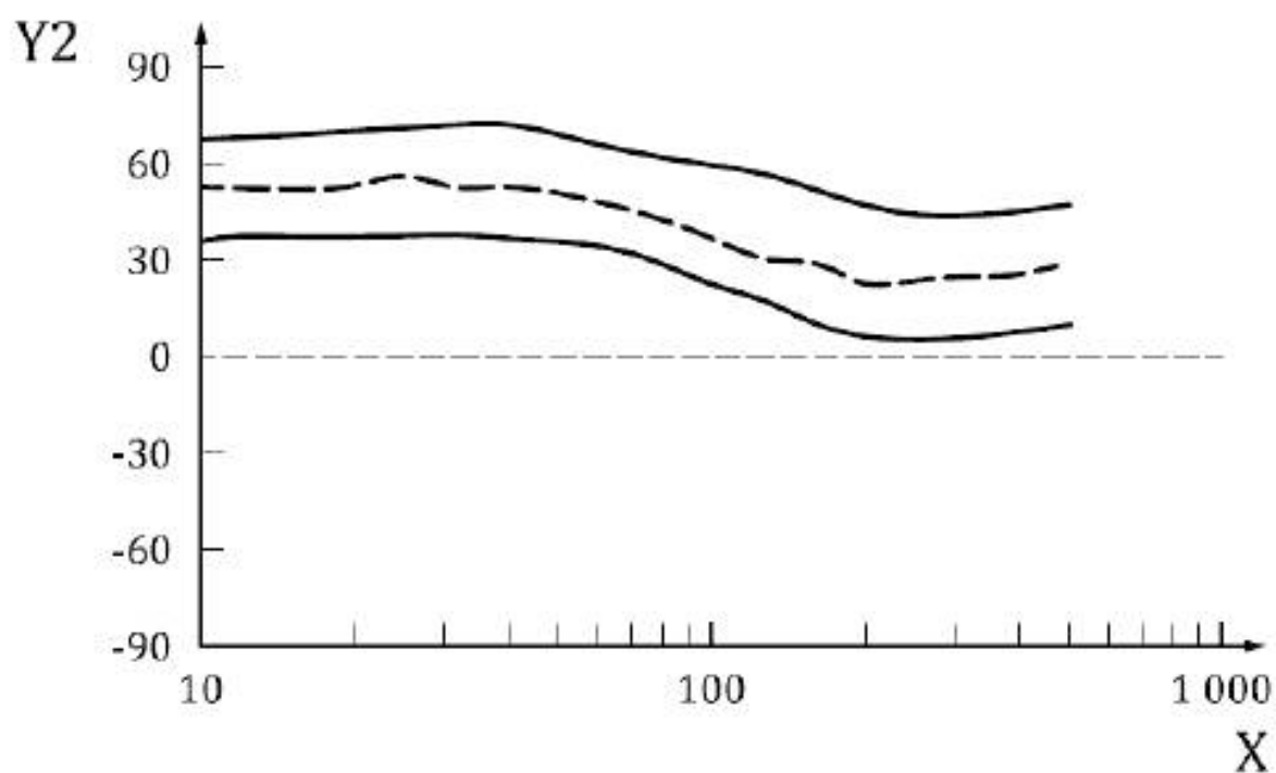
Рисунок 1 — Значения входного механического импеданса для системы «кисть — рука» в направлении x_b
