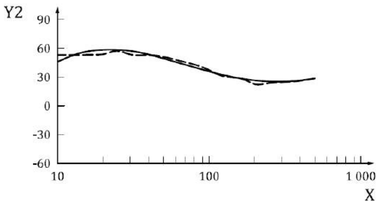
Рисунок С.2 — Сравнение результатов моделирования (сплошная линия) и опорных значений (пунктирная линия) механического импеданса системы «кисть — рука» в направлении x_0
