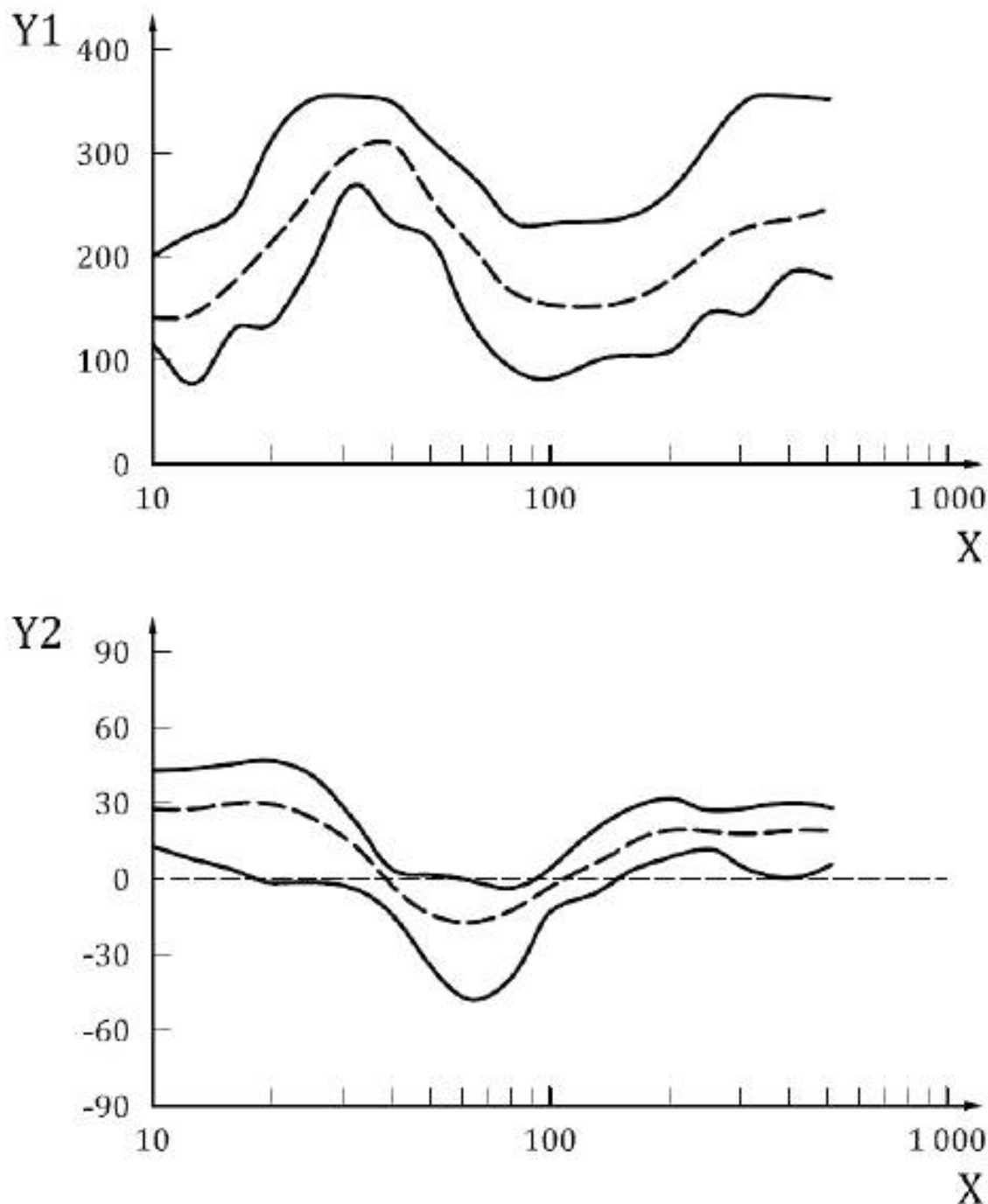
Рисунок 3 — Значения входного механического импеданса для системы «кисть — рука» в направлении z_0
