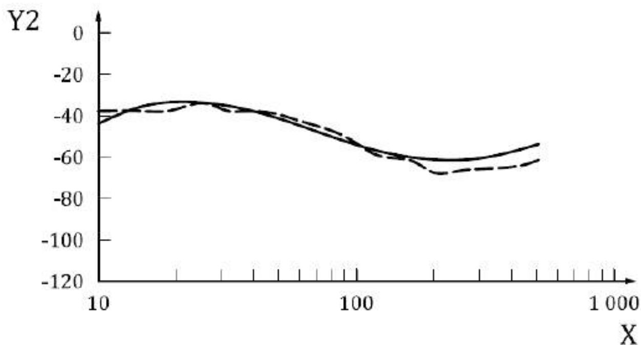
Рисунок В.2 — Сравнение результатов моделирования (сплошная линия) и опорных значений (пунктирная линия) эффективной массы системы «кисть — рука» в направлении x_1
