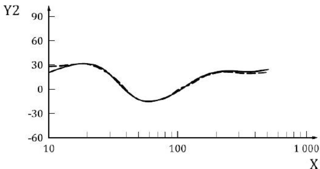
Рисунок С.4 — Сравнение результатов моделирования (сплошная линия) и опорных значений (пунктирная линия) механического импеданса системы «кисть — рука» в направлении z_x
