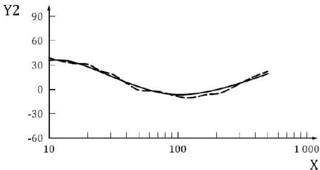
Рисунок С.3 — Сравнение результатов моделирования (сплошная линия) и опорных значений (пунктирная линия) механического импеданса системы «кисть — рука» в направлении y_z
