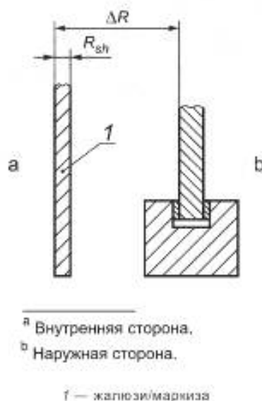
Рисунок 7 — Схема оконного блока с жалюзи или наружной маркизой
