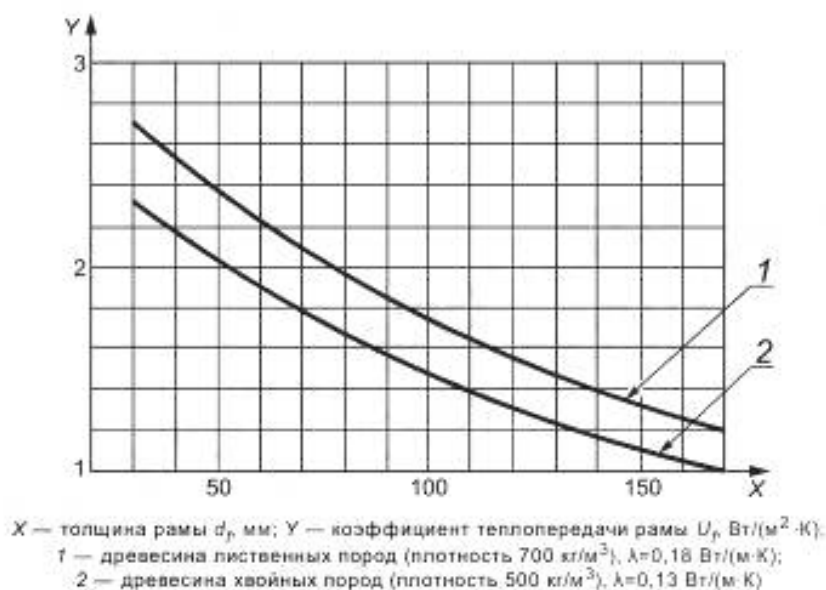
Рисунок F.2 — Коэффициент теплопередачи для деревянных и деревометаллических рам (см. рисунок F.3) в зависимости от их толщины d_f
