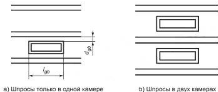
Рисунок G.3 — Схема двухкамерного стеклопакета со шпросами
