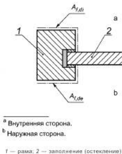
Рисунок 2 — Площади развертки рамы с внутренней и наружной сторон
