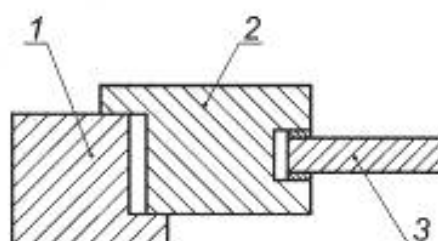
1 — коробка (неподвижная часть рамы); 2 — створка (подвижная часть рамы); 3 — остекление: одинарное или многослойное (стеклопакет)
