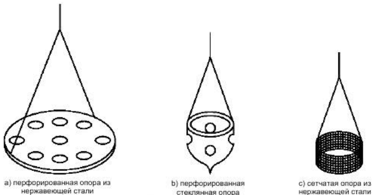
Рисунок 1 — Примеры опор образцов для испытаний
