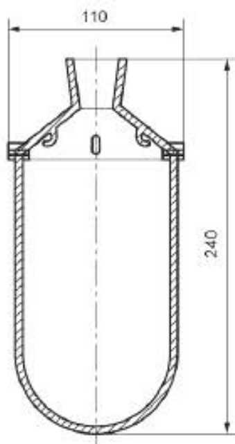
Рисунок 1 — Сосуд для проведения испытаний
