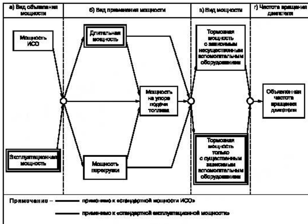
Рисунок 1 — Диаграмма, показывающая способы определения мощности
