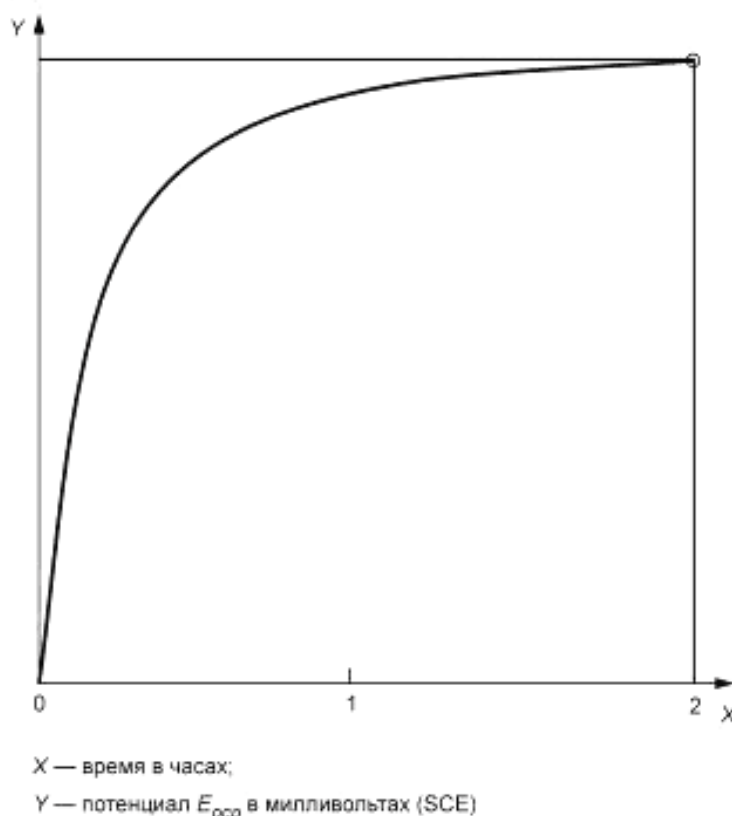
Рисунок 3 — Зависимость потенциала разомкнутой цепи от времени
