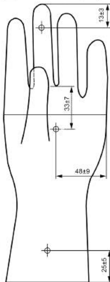
Рисунок 2 — Точки измерения толщины
