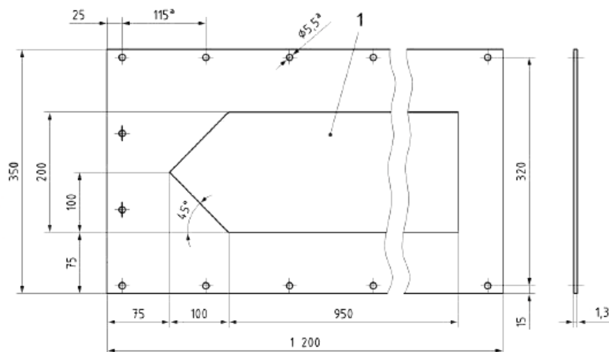
Рисунок 7 – Сборный узел регулируемого выходного отверстия. Пластина апертуры (нержавеющая сталь)
