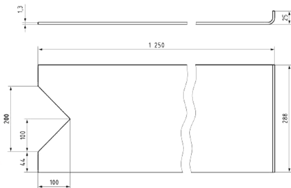
Рисунок 8 - Сборный узел регулируемого выходного отверстия. Задвижка (нержавеющая сталь)
