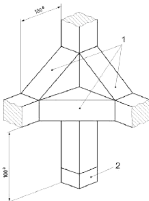
Рисунок 2 - Испытательная камера. Детали крепления пленки
