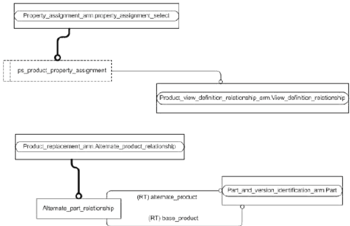
Рисунок С.2 — Представление ПЗМ на уровне объектов в формате EXPRESS-G
