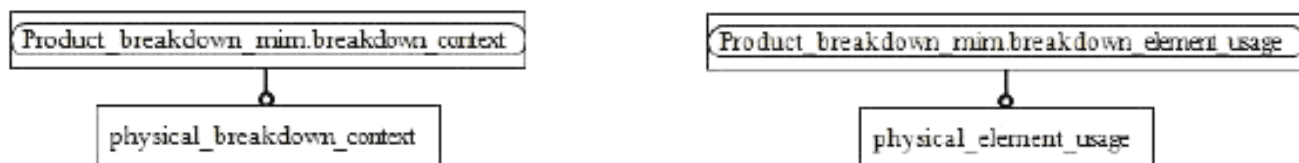
Рисунок D.2 – Представление IMM на уровне объектов в формате EXPRESS-G
