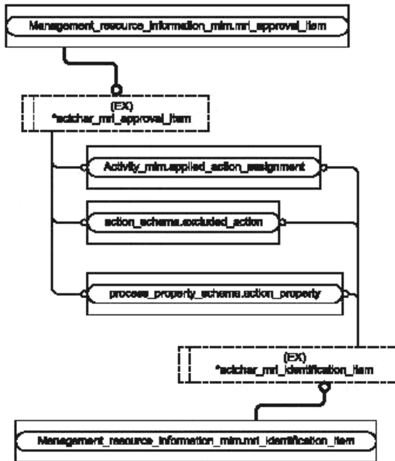
Рисунок D.3 — Представление IMM на уровне объектов в формате EXPRESS-G (диаграмма 2 из 6)
