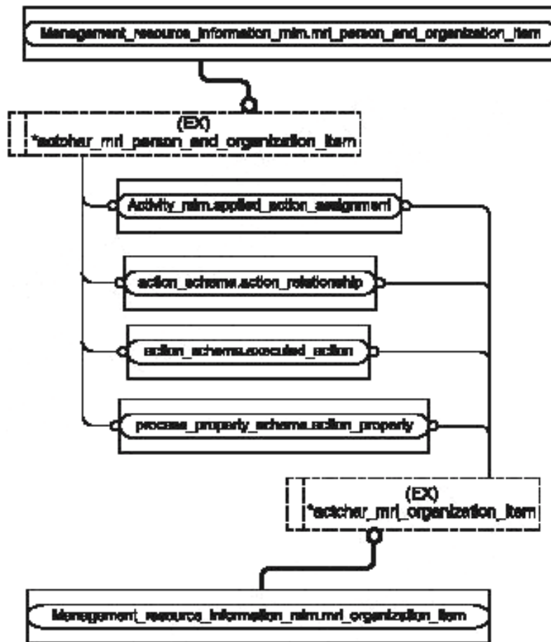
Рисунок D.5 — Представление IMM на уровне объектов в формате EXPRESS-G (диаграмма 4 из 6)
