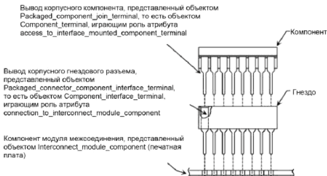
Рисунок 3 — Вывод корпусного компонента, представленный объектом Packaged_component_join_terminal
