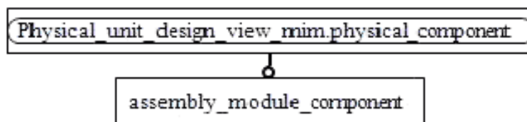
Рисунок D.2 – Представление IMM на уровне объектов в формате EXPRESS-G
