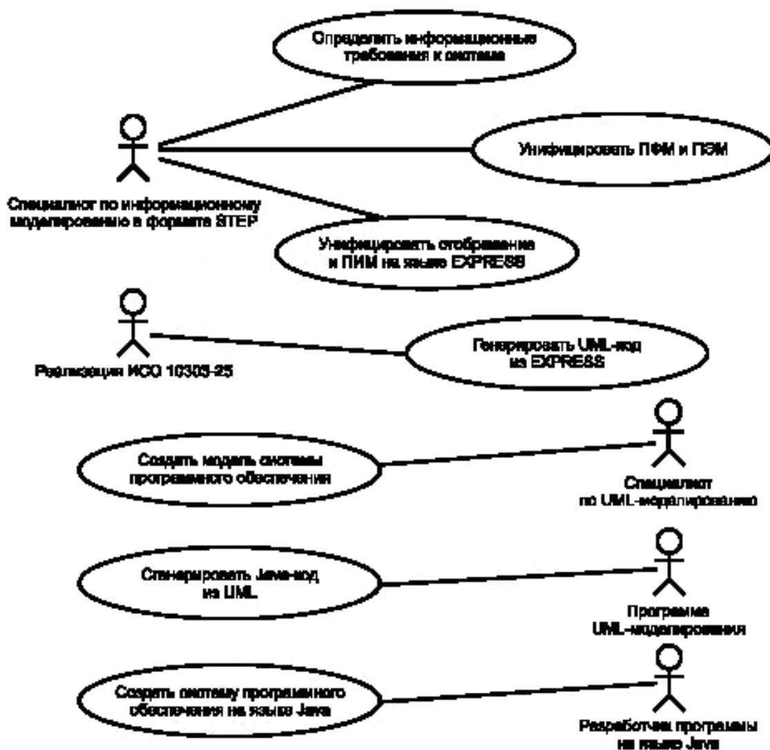
Рисунок 1 — Реализация прикладного протокола
