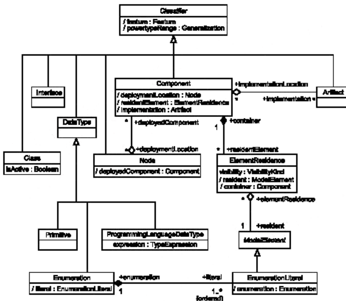
Рисунок D.3 — Главный пакет — Классификаторы (рисунок 5-5 из [4])
