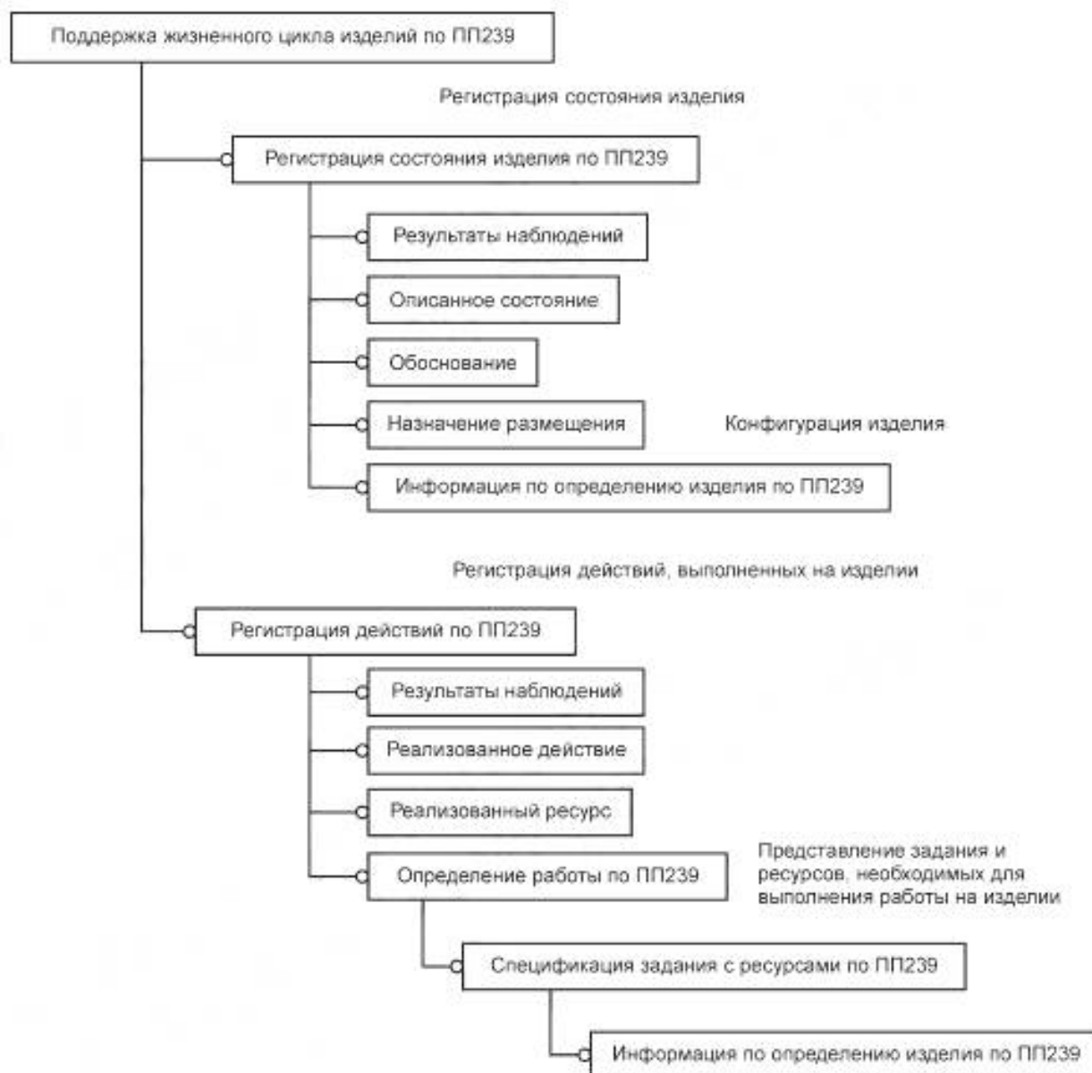
Рисунок 3 — Основная часть иерархии модулей
