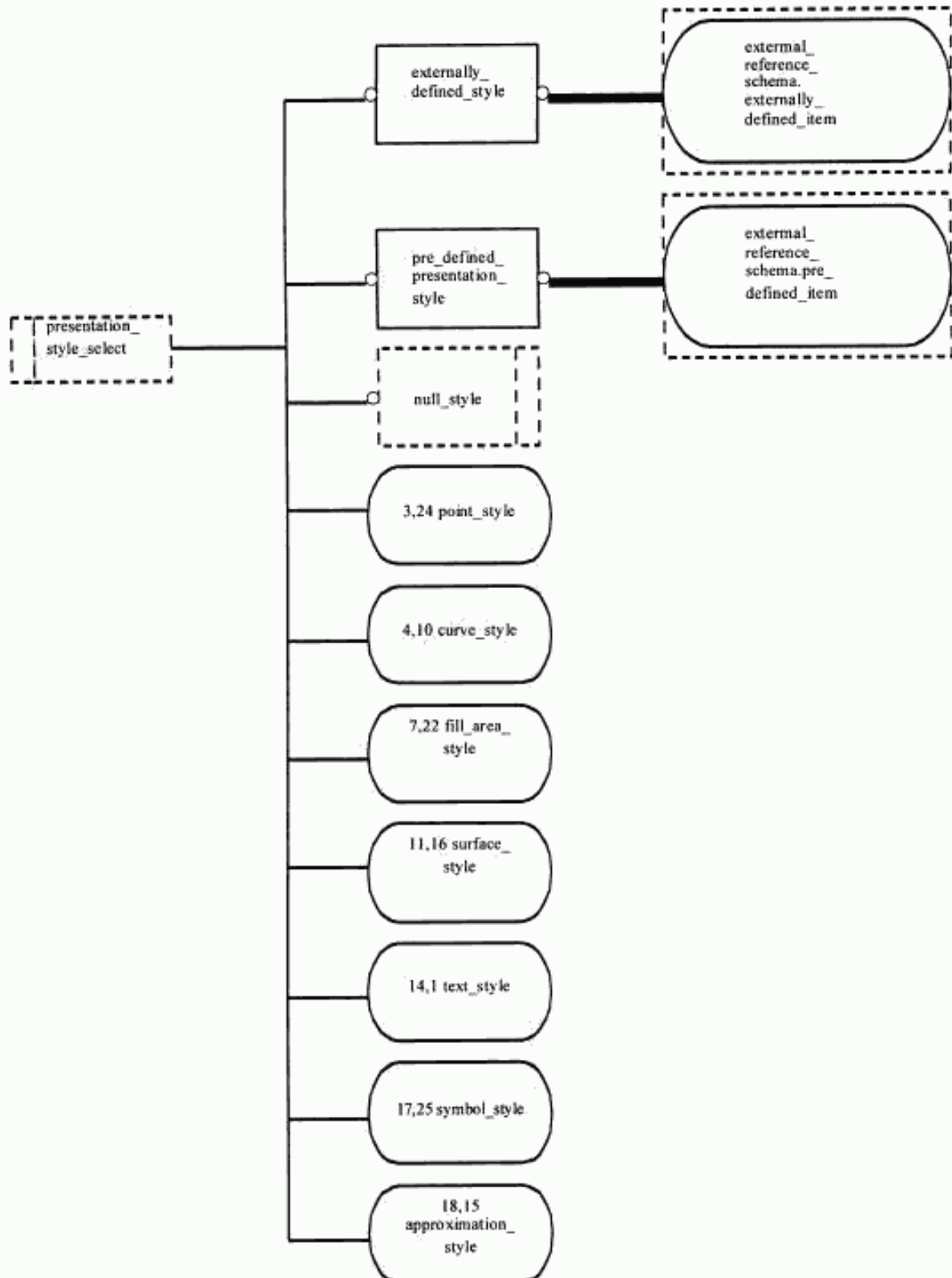
Рисунок E.18 — EXPRESS-G диаграмма presentation_appearance_schema 2 из 21
