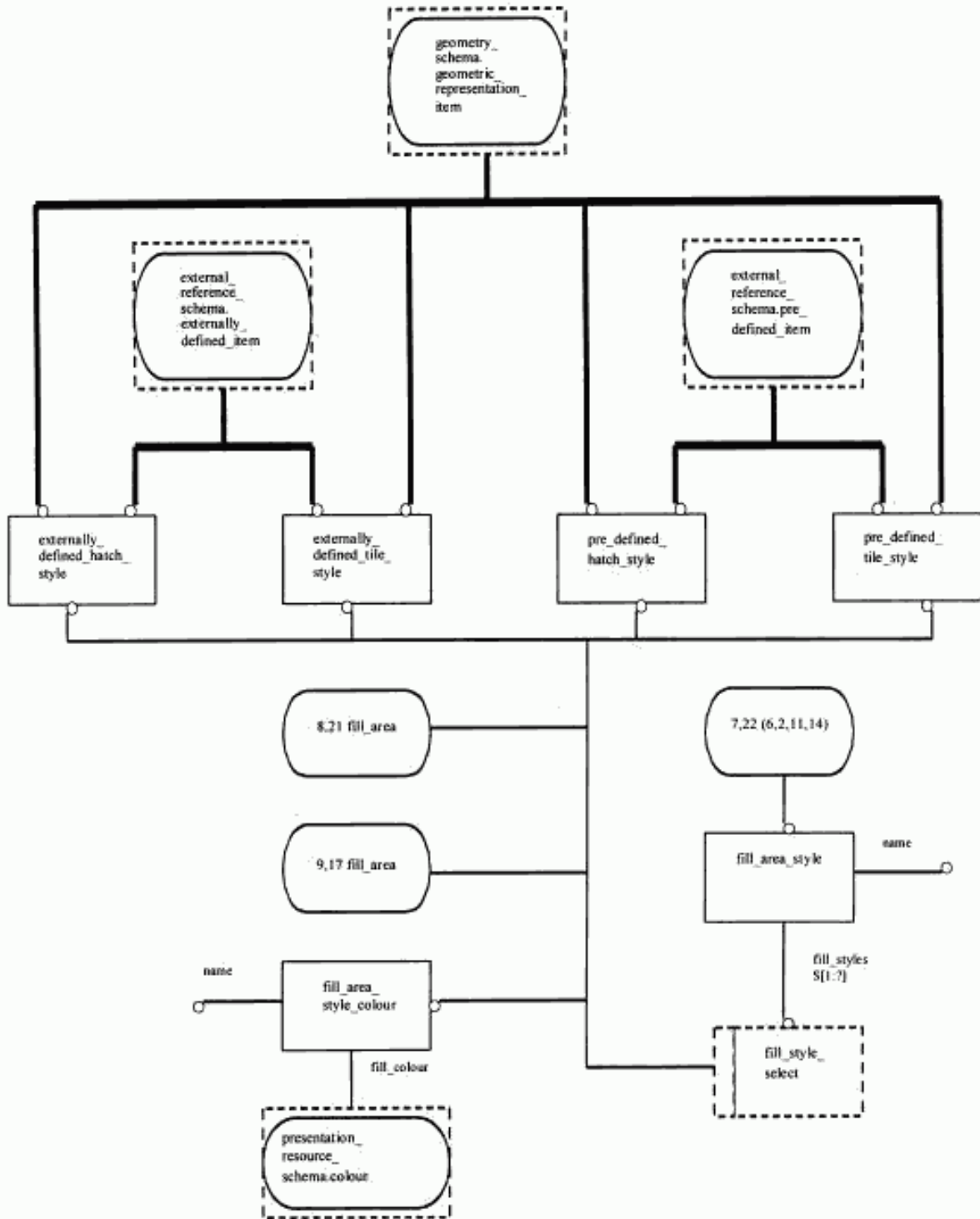
Рисунок E.23 — EXPRESS-G диаграмма presentation_appearance_schema 7 из 21
