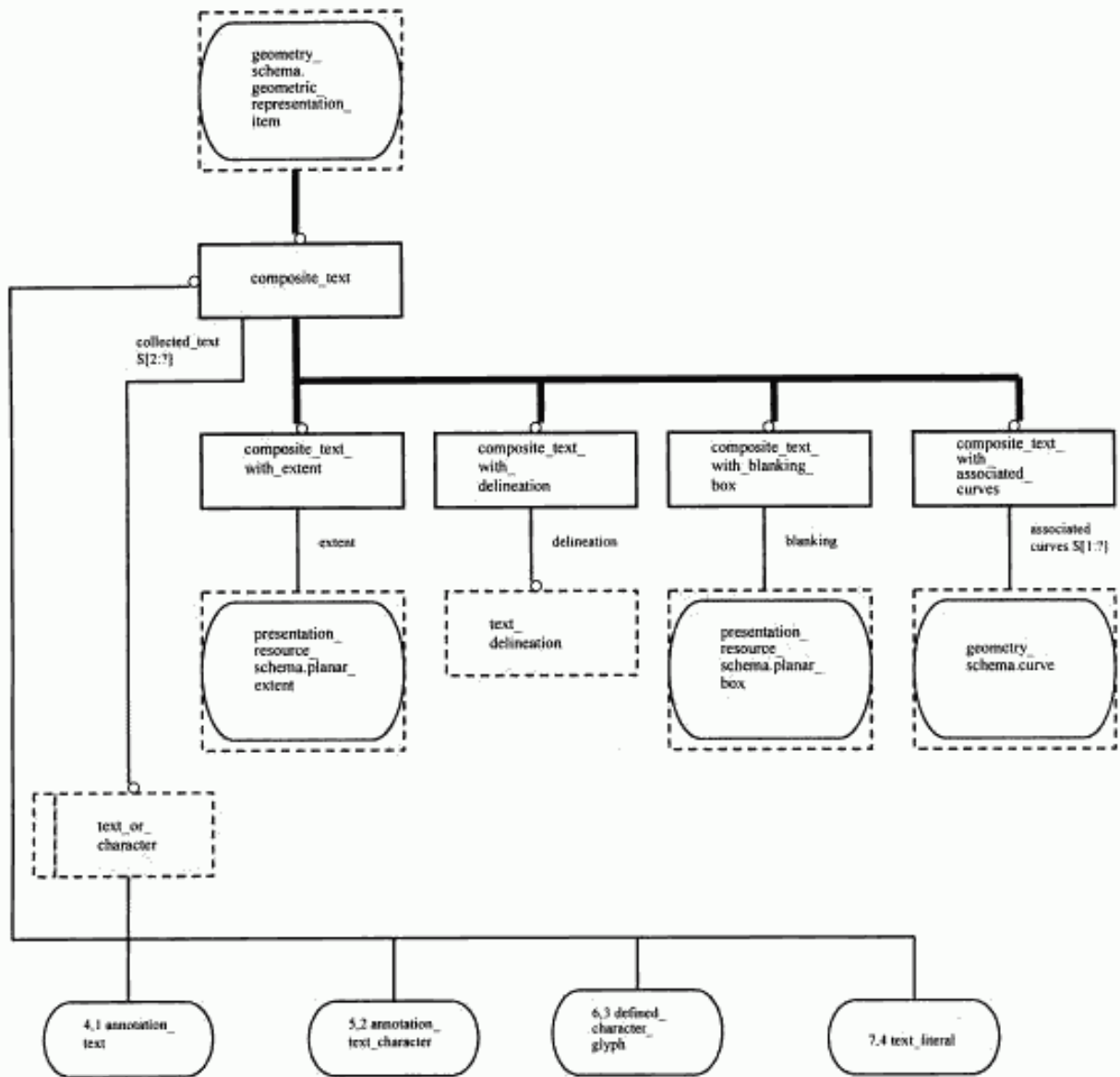
Рисунок E.15 — EXPRESS-G диаграмма presentation_definition_schema 8 из 9
