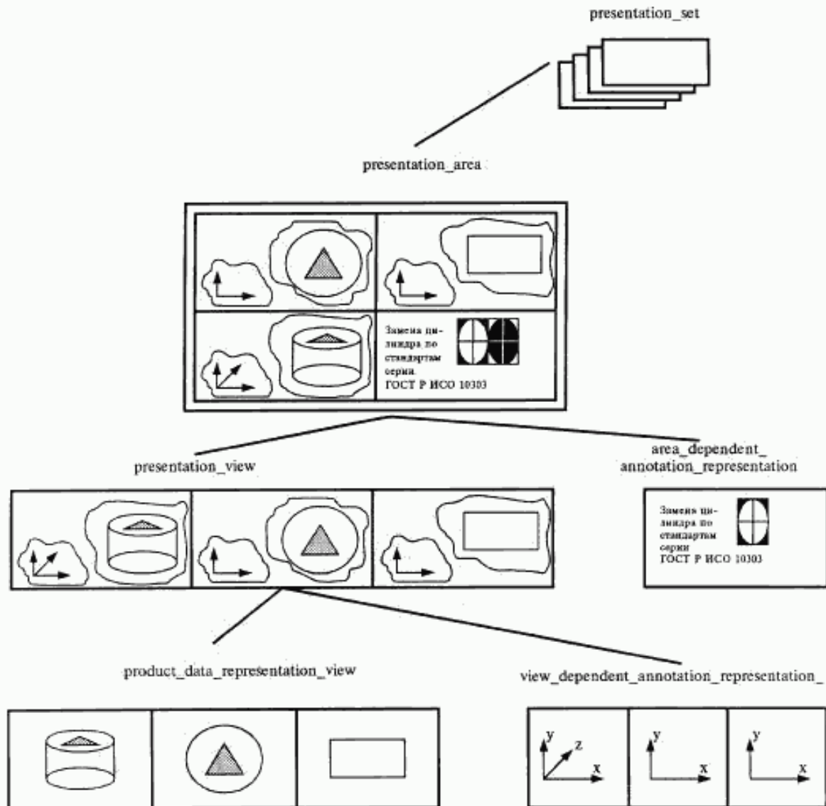
Рисунок 2 — Пример иерархии представления
