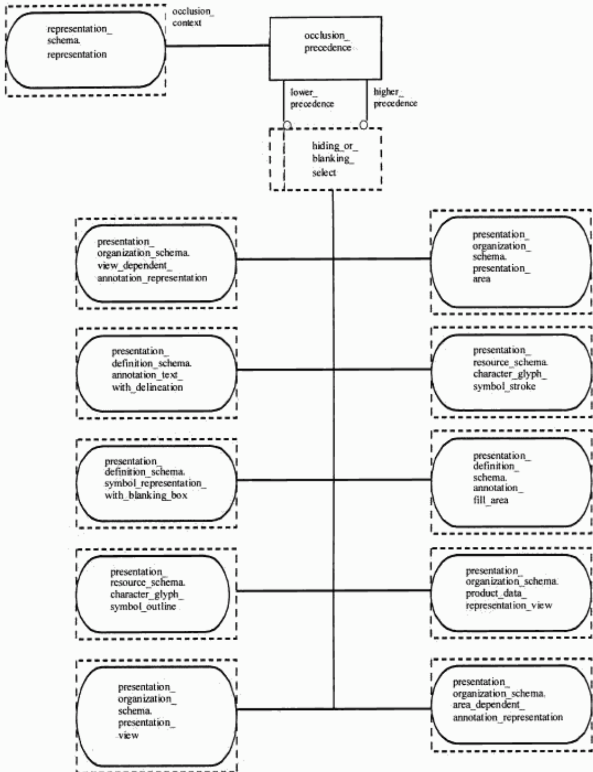
Рисунок E.36 — EXPRESS-G диаграмма presentation_appearance_schema 20 из 21
