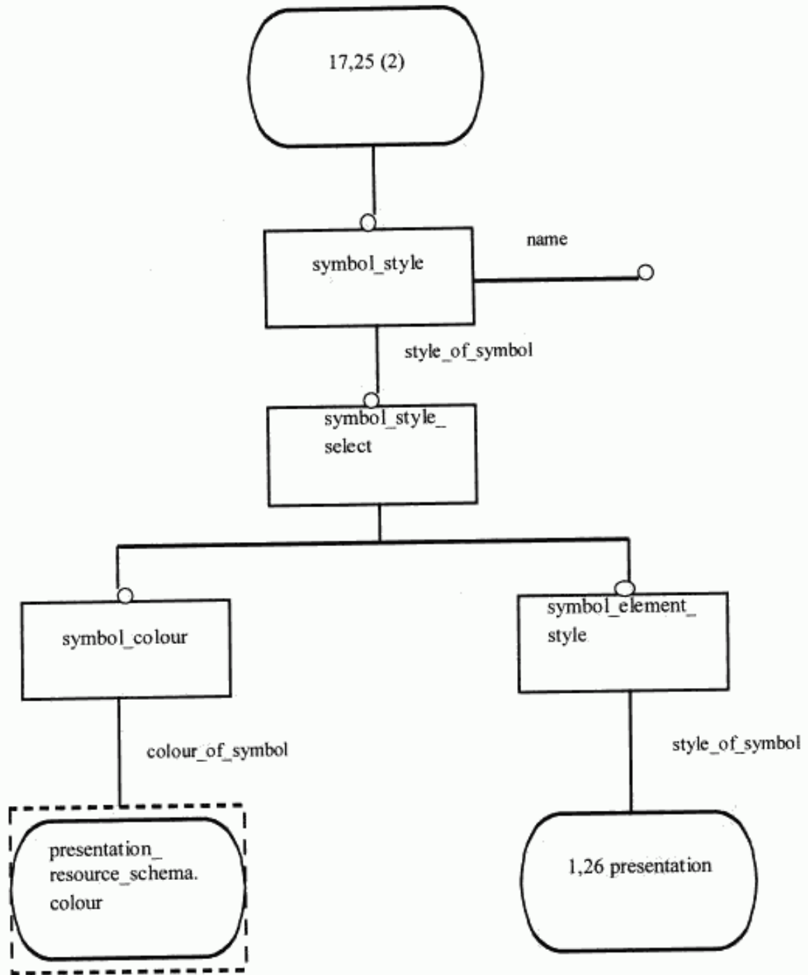
Рисунок Е.33 — EXPRESS-G диаграмма presentation_appearance_schema 17 из 21
