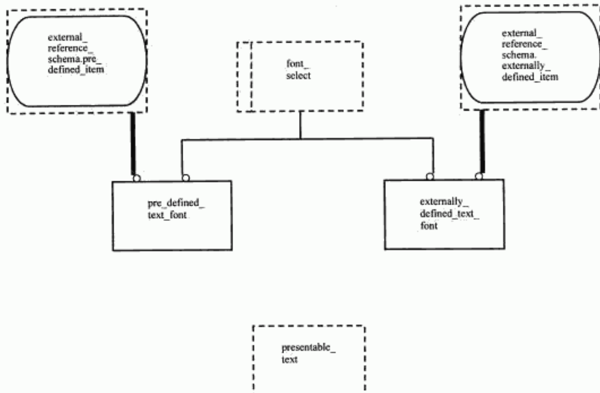
Рисунок E.40 — EXPRESS-G диаграмма presentation_resource_schema 3 из 5
