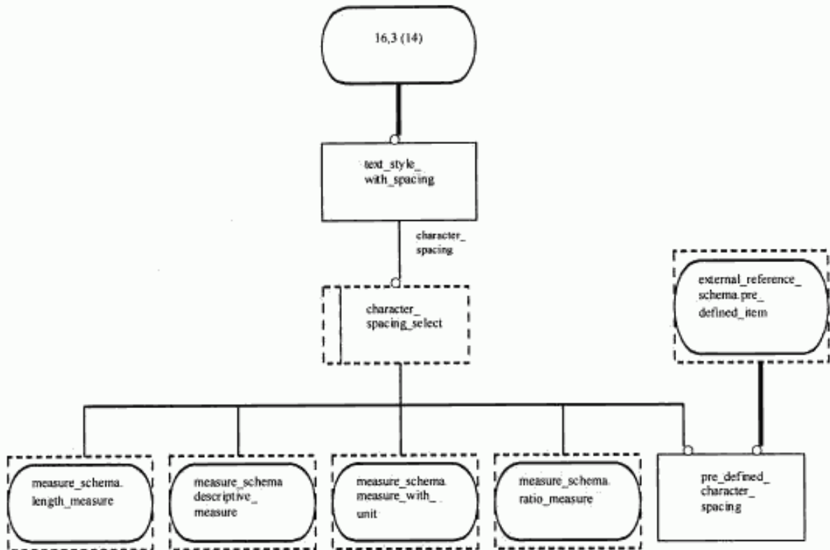
Рисунок E.32 — EXPRESS-G диаграмма presentation_appearance_schema 16 из 21
