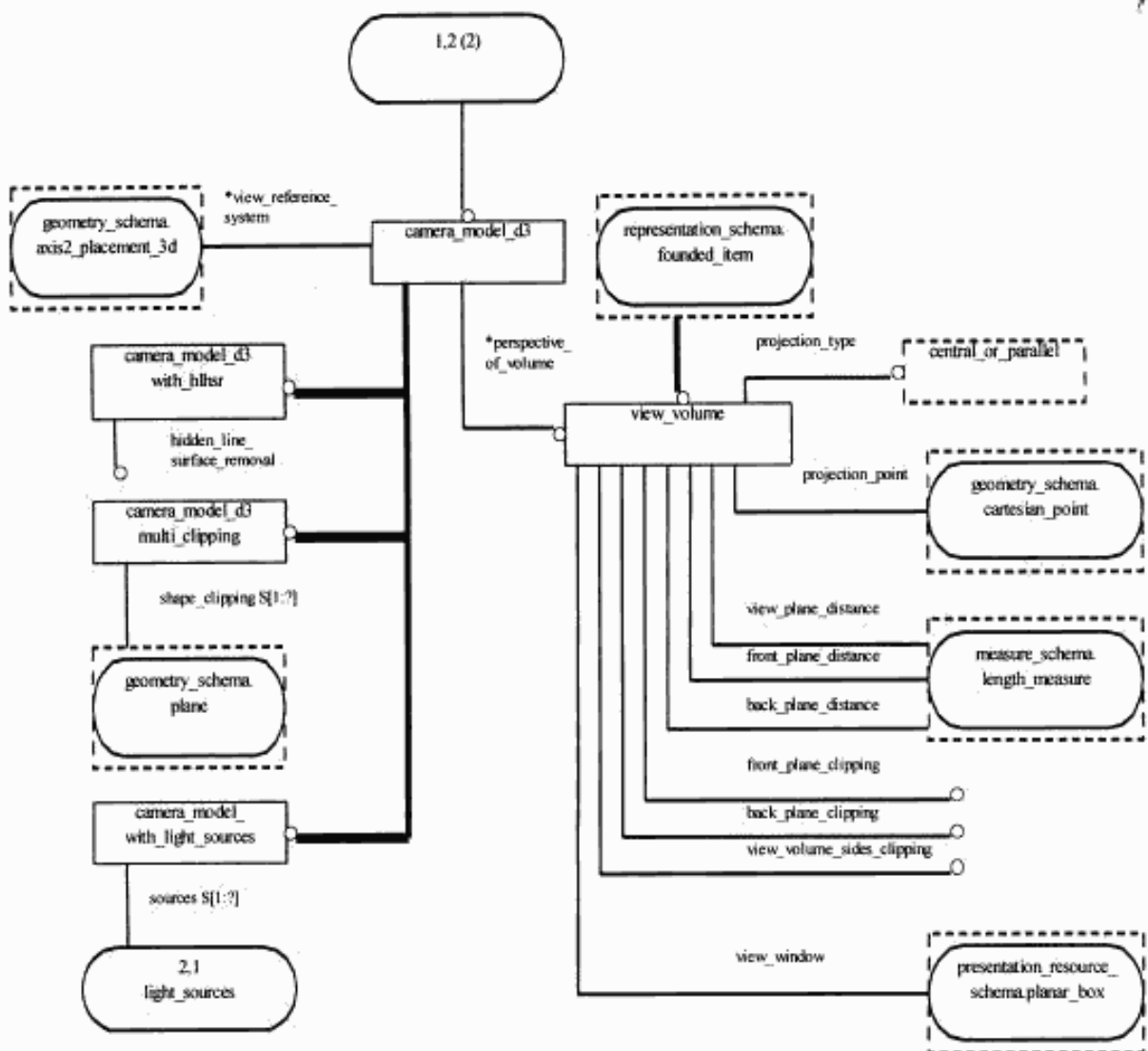
Рисунок Е.4 — EXPRESS-G диаграмма presentation_organization_schema 4 из 7
