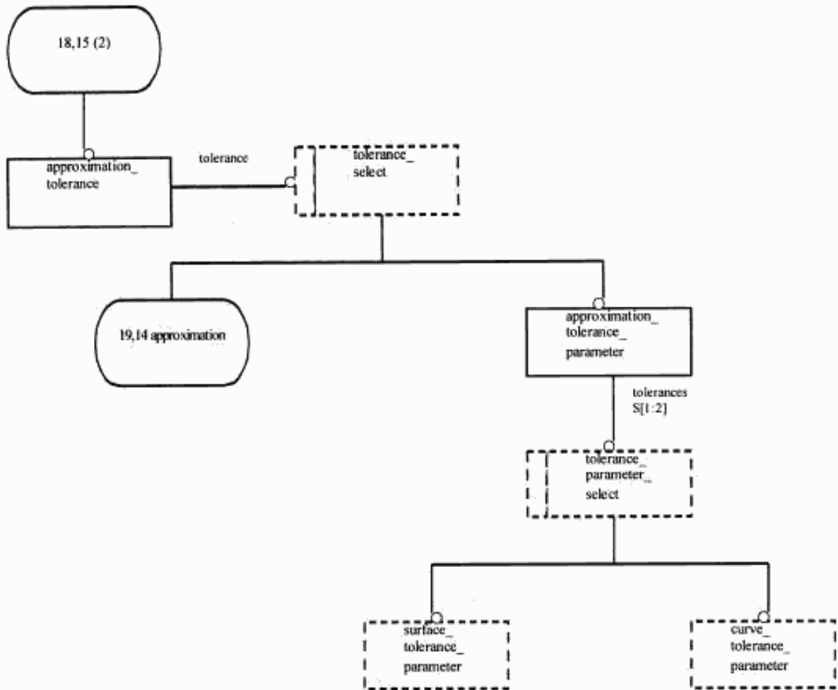
Рисунок E.34 — EXPRESS-G диаграмма presentation_appearance_schema 18 из 21
