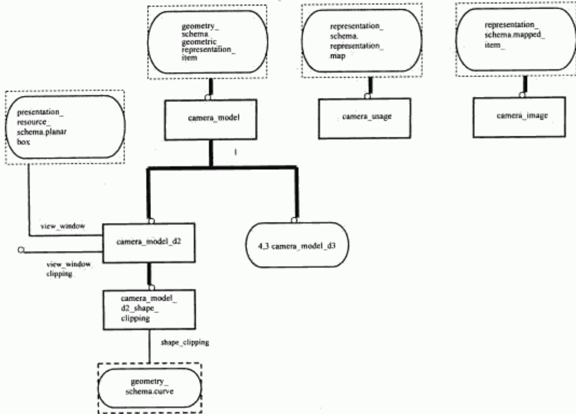
Рисунок E.3 — EXPRESS-G диаграмма presentation_organization_schema 3 из 7
