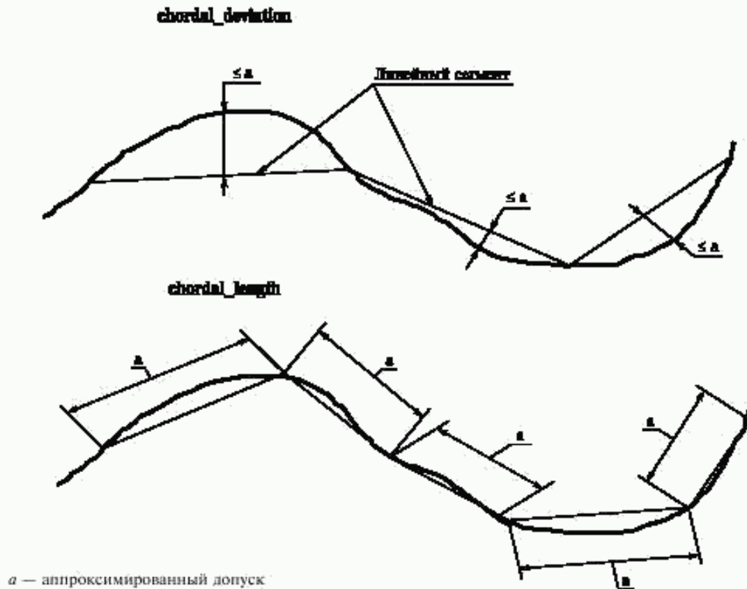
Рисунок 18 — Отклонение и длина хорды
