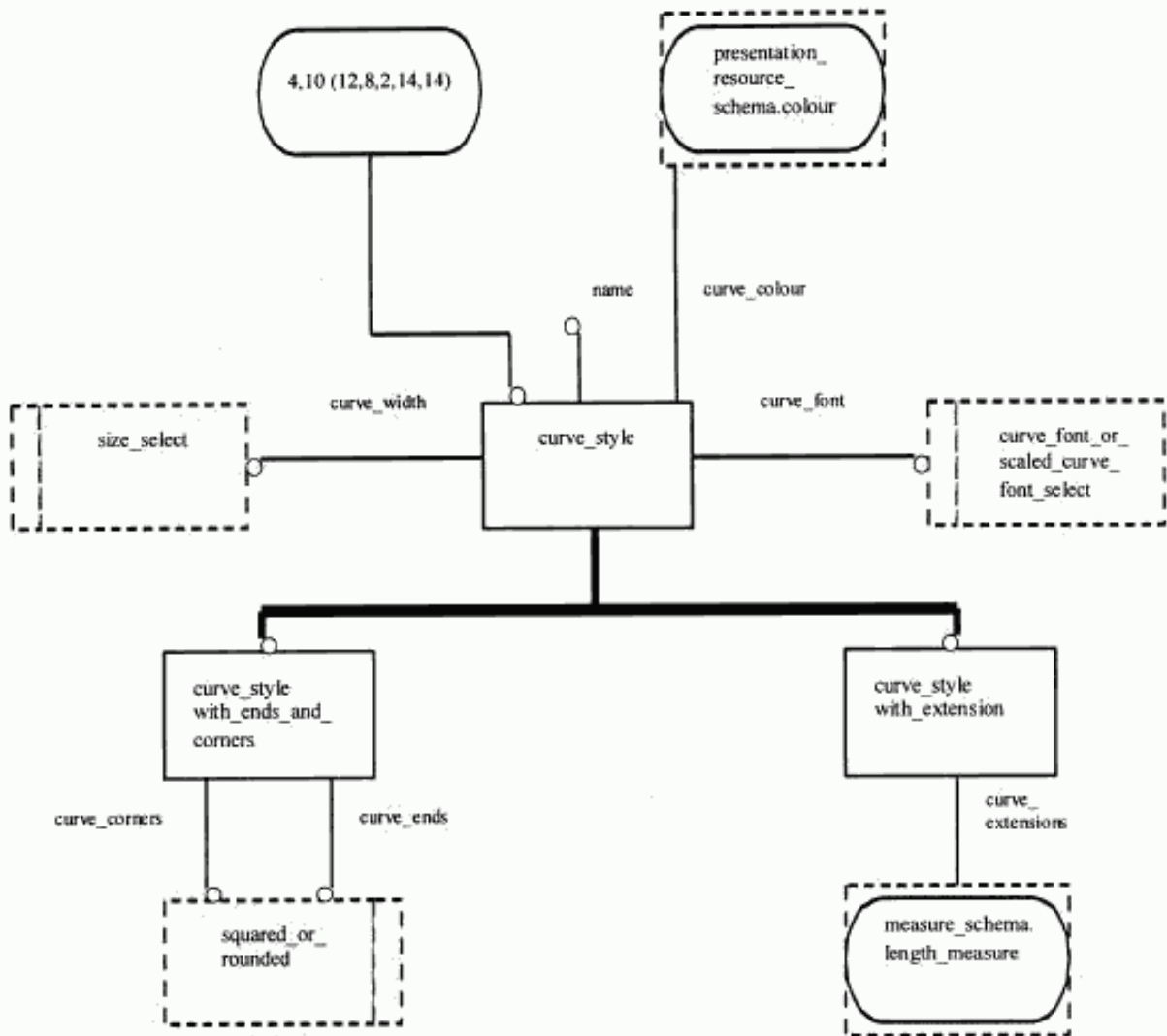
Рисунок E.20 — EXPRESS-G диаграмма presentation_appearance_schema 4 из 21
