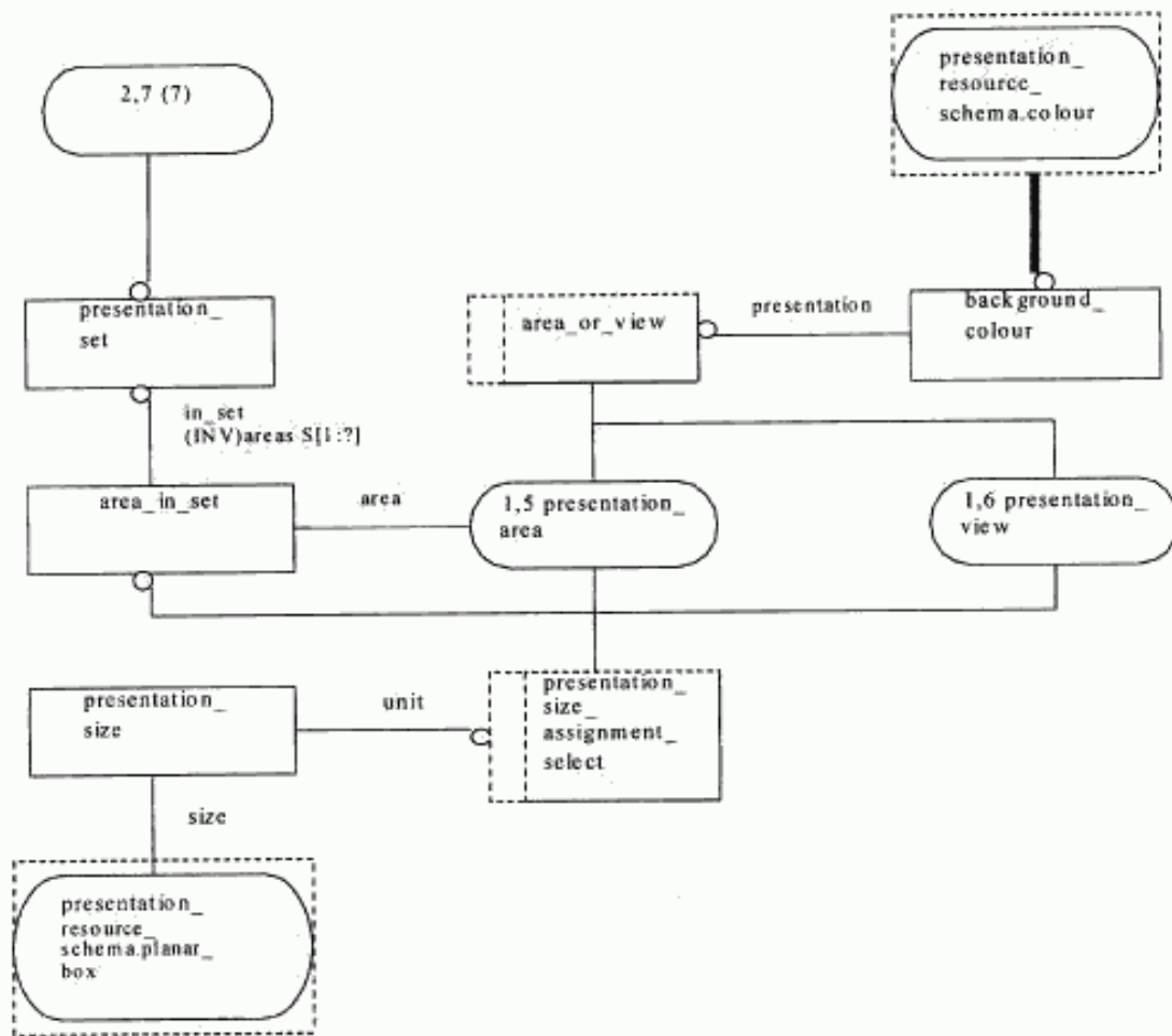
Рисунок E.2 — EXPRESS-G диаграмма presentation_organization_schema 2 из 7
