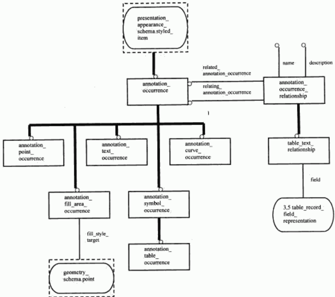
Рисунок E.16 — EXPRESS-G диаграмма presentation_definition_schema 9 из 9
