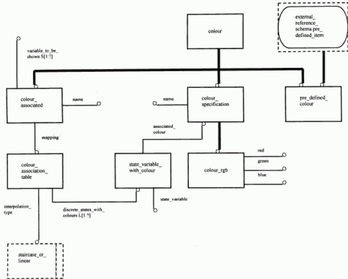
Рисунок E.41 — EXPRESS-G диаграмма presentation_resource_schema 4 из 5
