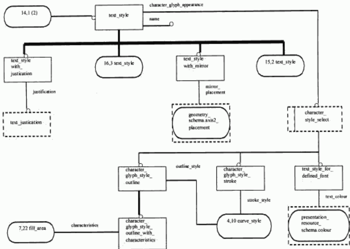
Рисунок E.30 — EXPRESS-G диаграмма presentation_appearance_schema 14 из 21
