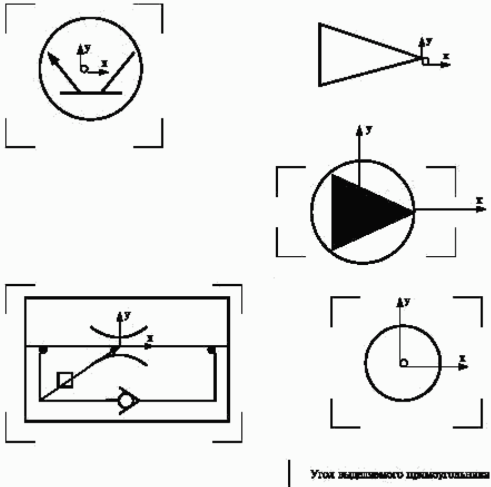
Рисунок 15 — Примеры аннотируемых символов
