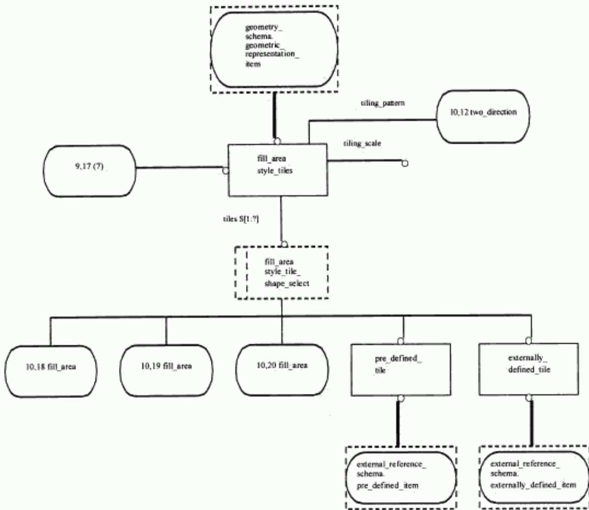
Рисунок E.25 — EXPRESS-G диаграмма presentation_appearance_schema 9 из 21
