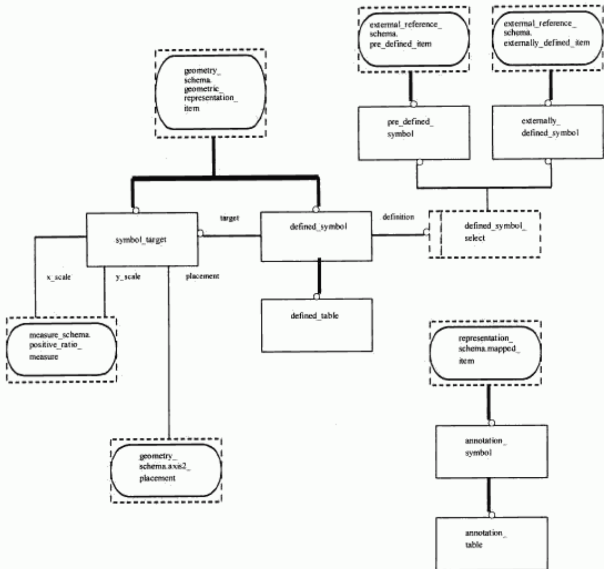
Рисунок E.9 — EXPRESS-G диаграмма presentation_definition_schema 2 из 9
