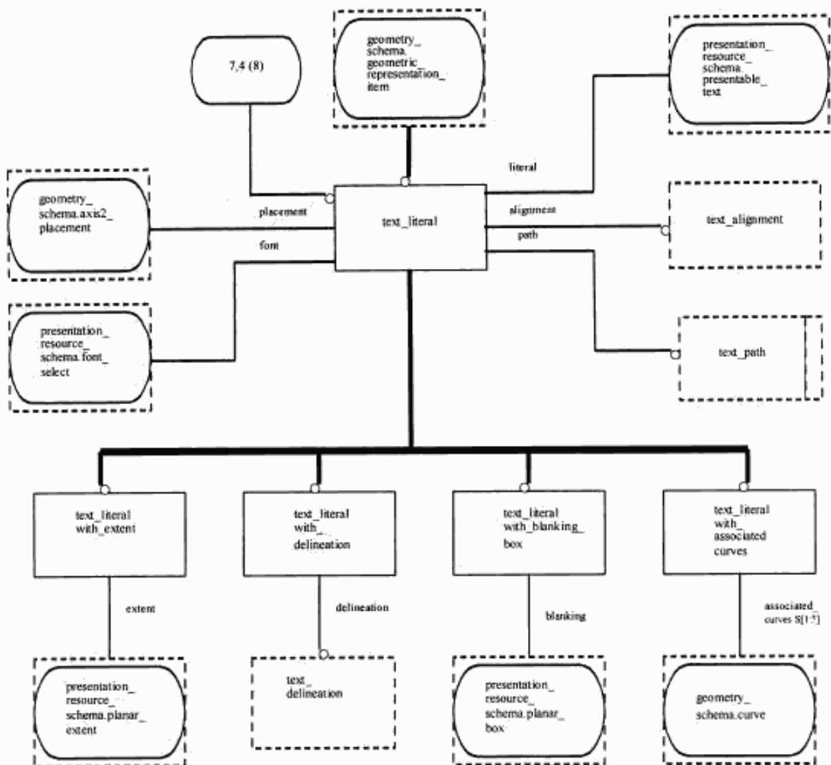
Рисунок E.14 — EXPRESS-G диаграмма presentation_definition_schema 7 из 9
