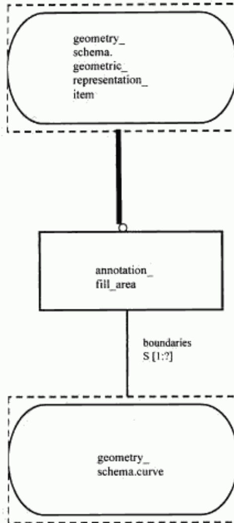
Рисунок E.8 — EXPRESS-G диаграмма presentation_definition_schema 1 из 9
