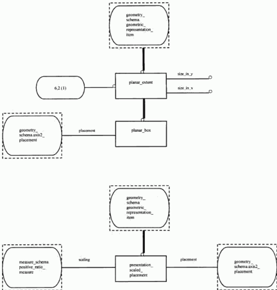
Рисунок E.42 — EXPRESS-G диаграмма presentation_resource_schema 5 из 5
