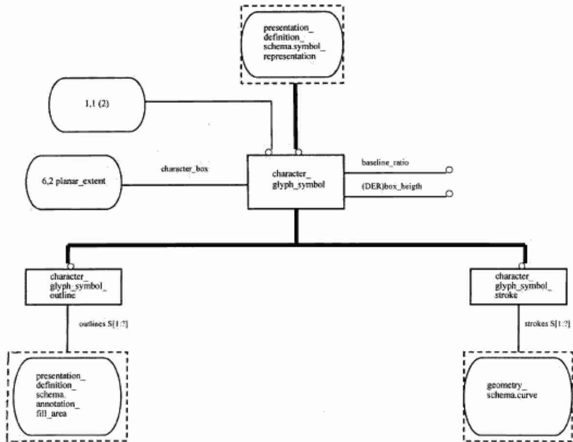
Рисунок Е.38 — EXPRESS-G диаграмма presentation_resource_schema 1 из 5
