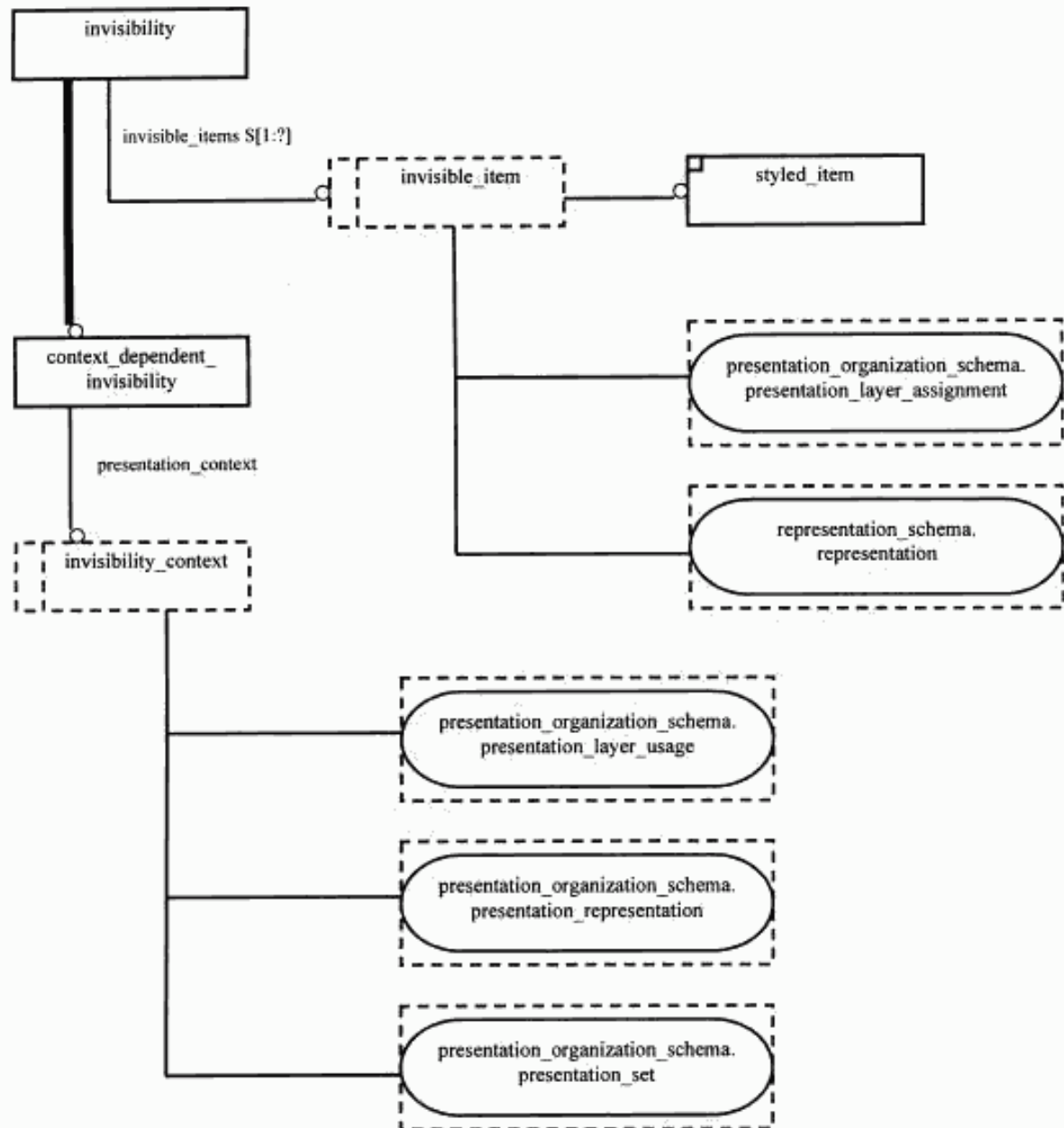
Рисунок E.37 — EXPRESS-G диаграмма presentation_appearance_schema 21 из 21
