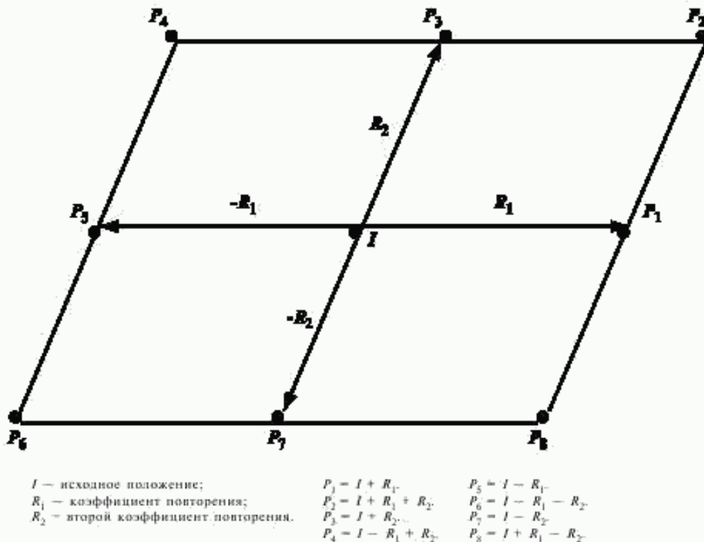
Рисунок 23 — Коэффициент повтора двумерного изображения
