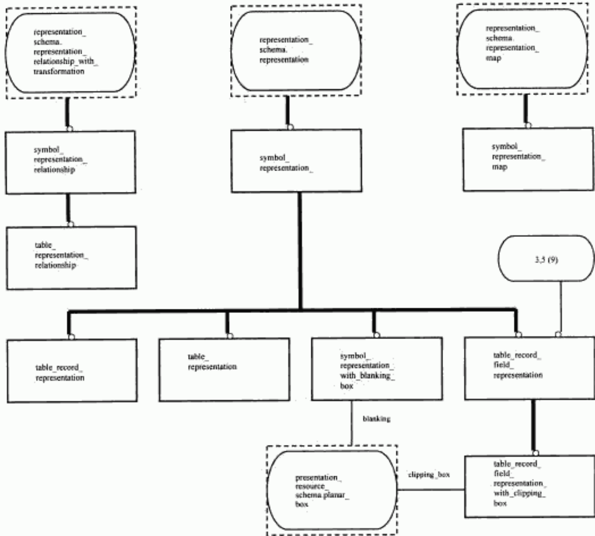
Рисунок E.10 — EXPRESS-G диаграмма presentation_definition_schema 3 из 9
