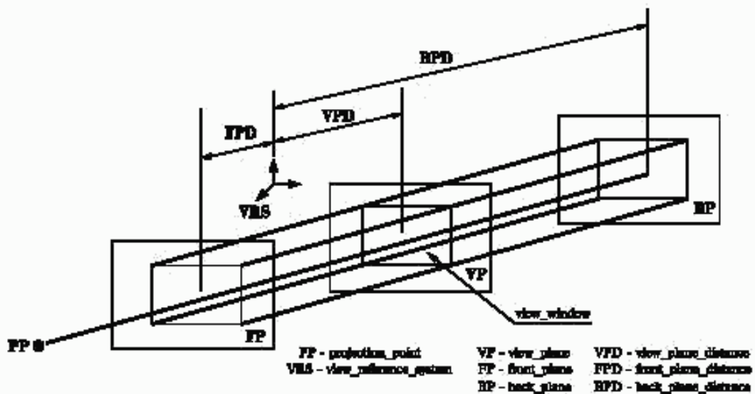
Рисунок 8 — Вид объема, тип проекции — PARALLEL
