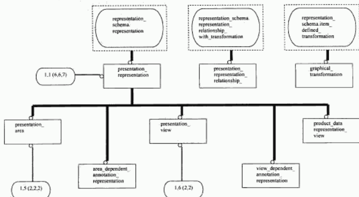
Рисунок Е.1 — EXPRESS-G диаграмма presentation_organization_schema 1 из 7
