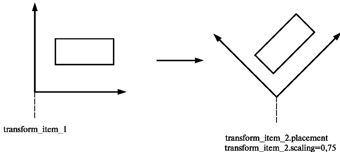
Рисунок 5 — Графическое преобразование
