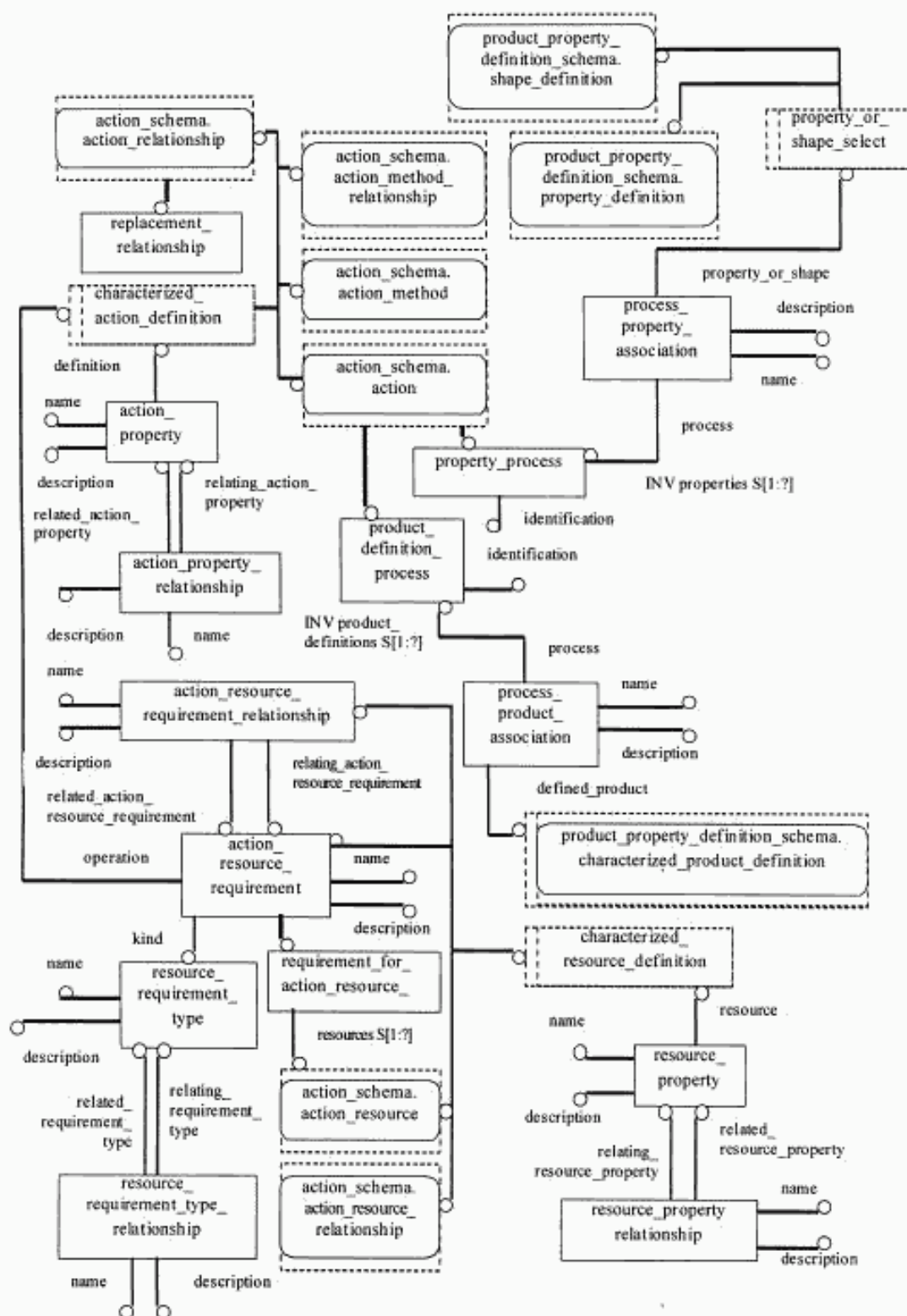
Рисунок D.2 — product_concept_schema — EXPRESS-G диаграмма 1 из 1
