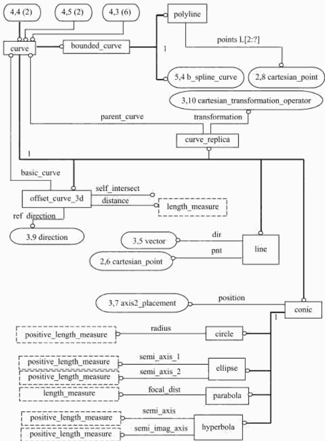
Рисунок С.4 — alc_edge_based_wireframe — EXPRESS-G диаграмма 4 из 6
