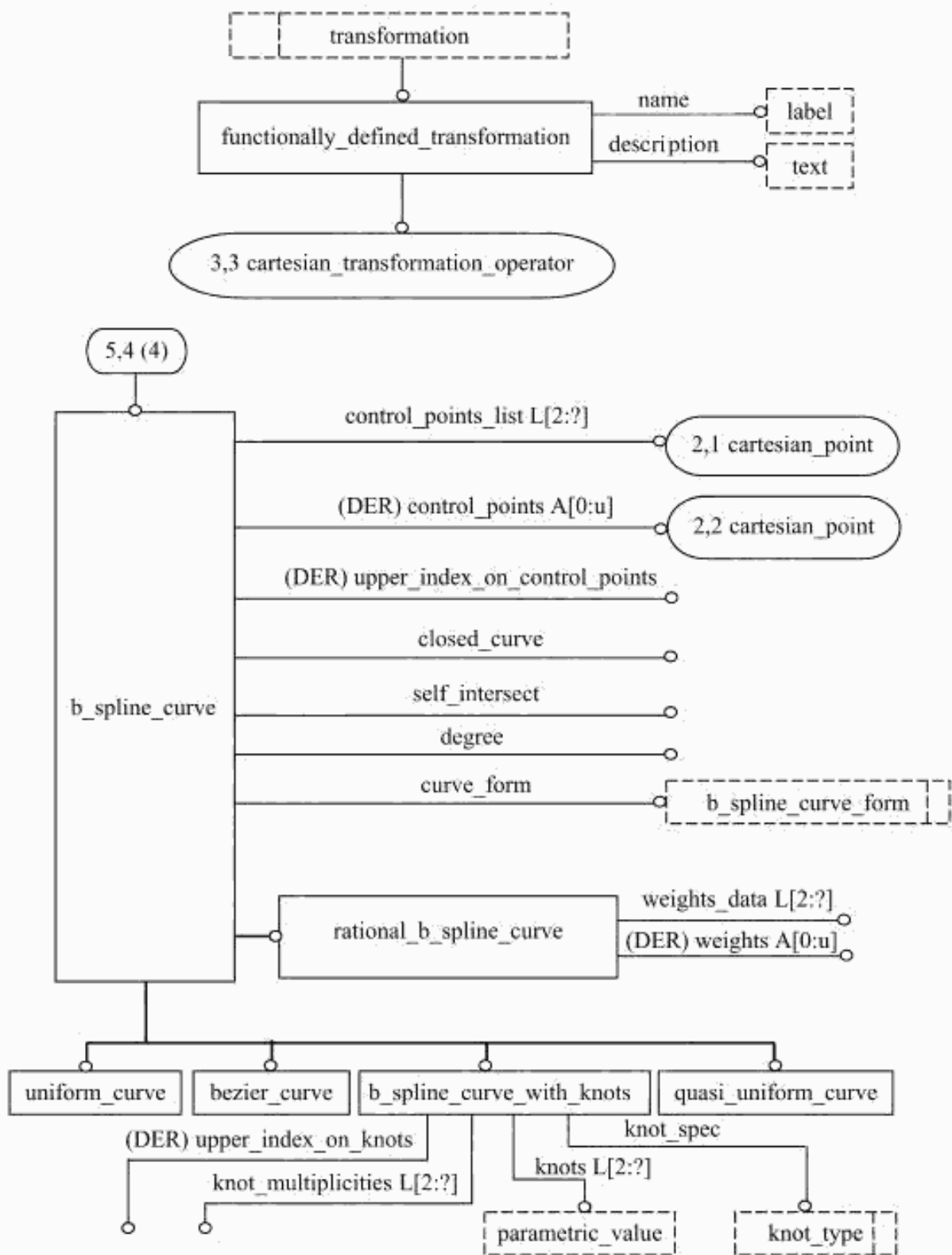
Рисунок С.5 — alc_edge_based_wireframe — EXPRESS-G диаграмма 5 из 6
