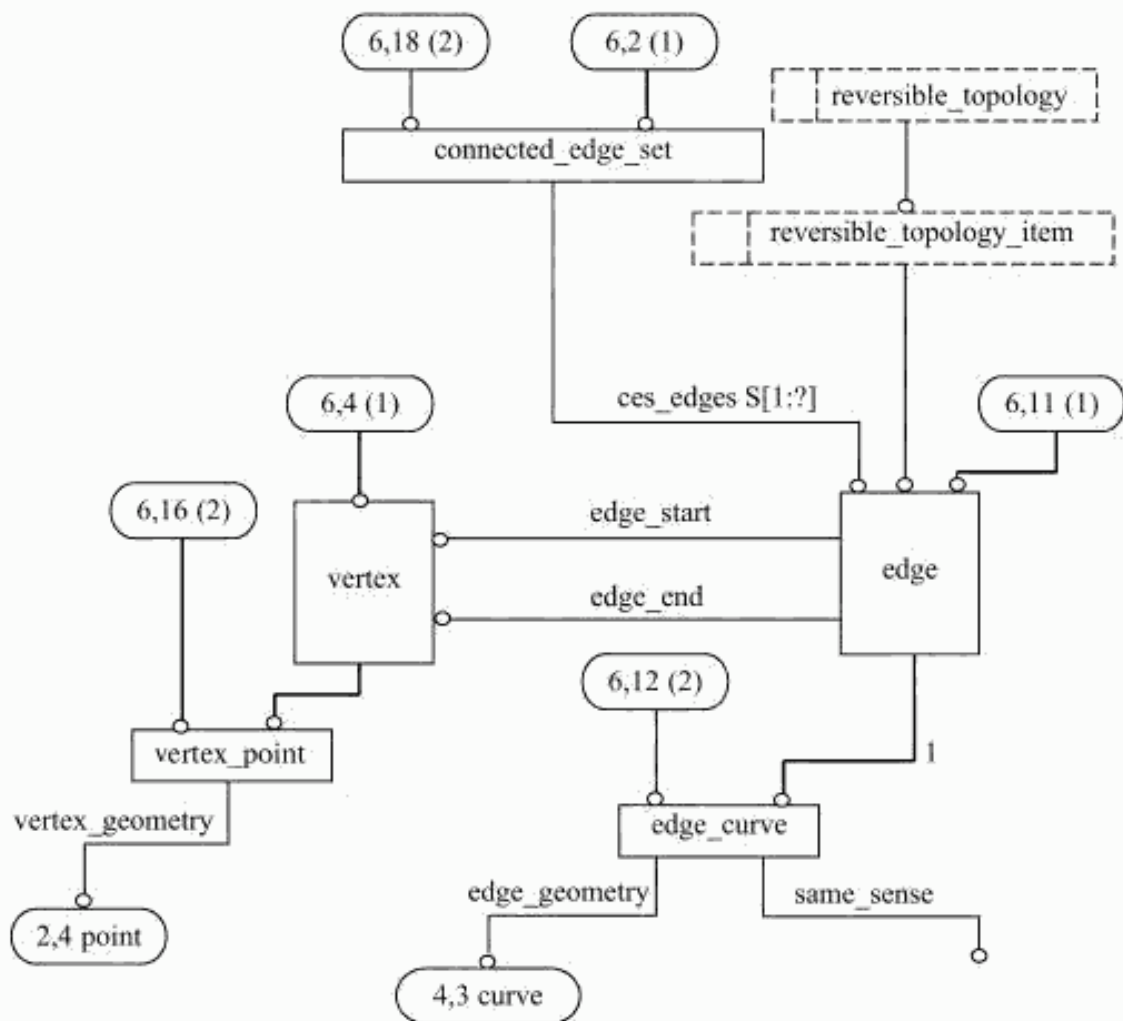
Рисунок С.6 — aic_edge_based_wireframe — EXPRESS-G диаграмма 6 из 6
