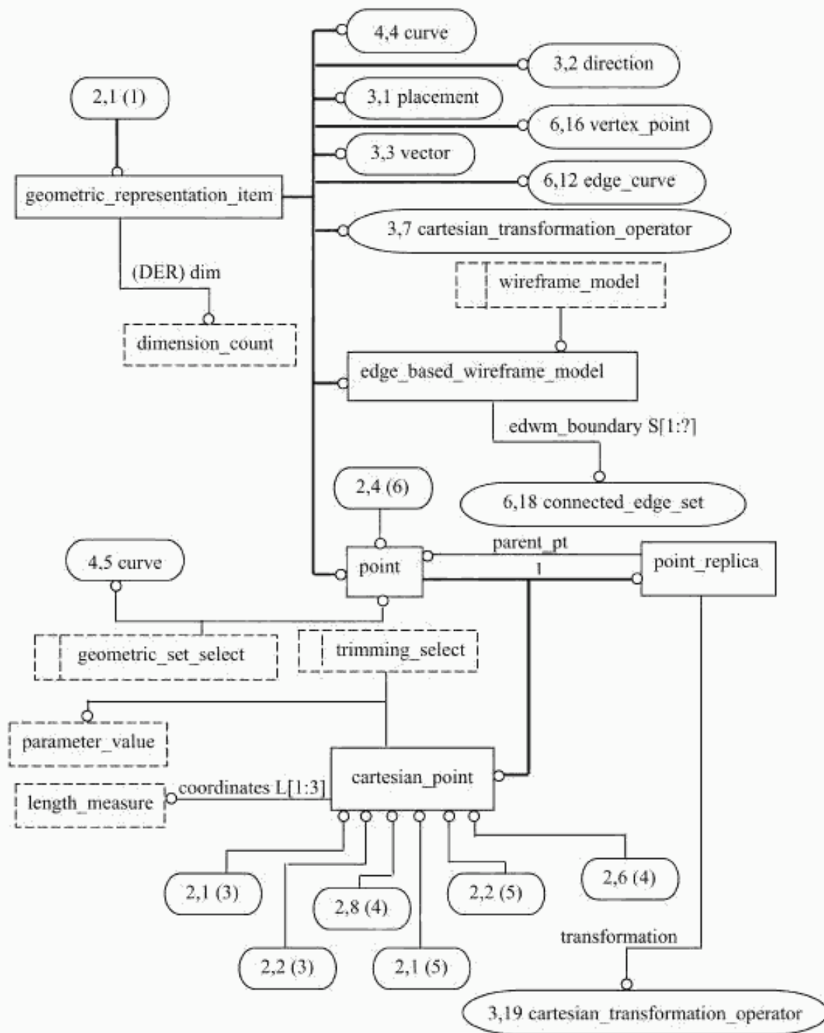
Рисунок С.2 — a1c_edge_based_wireframe — EXPRESS-G диаграмма 2 из 6
