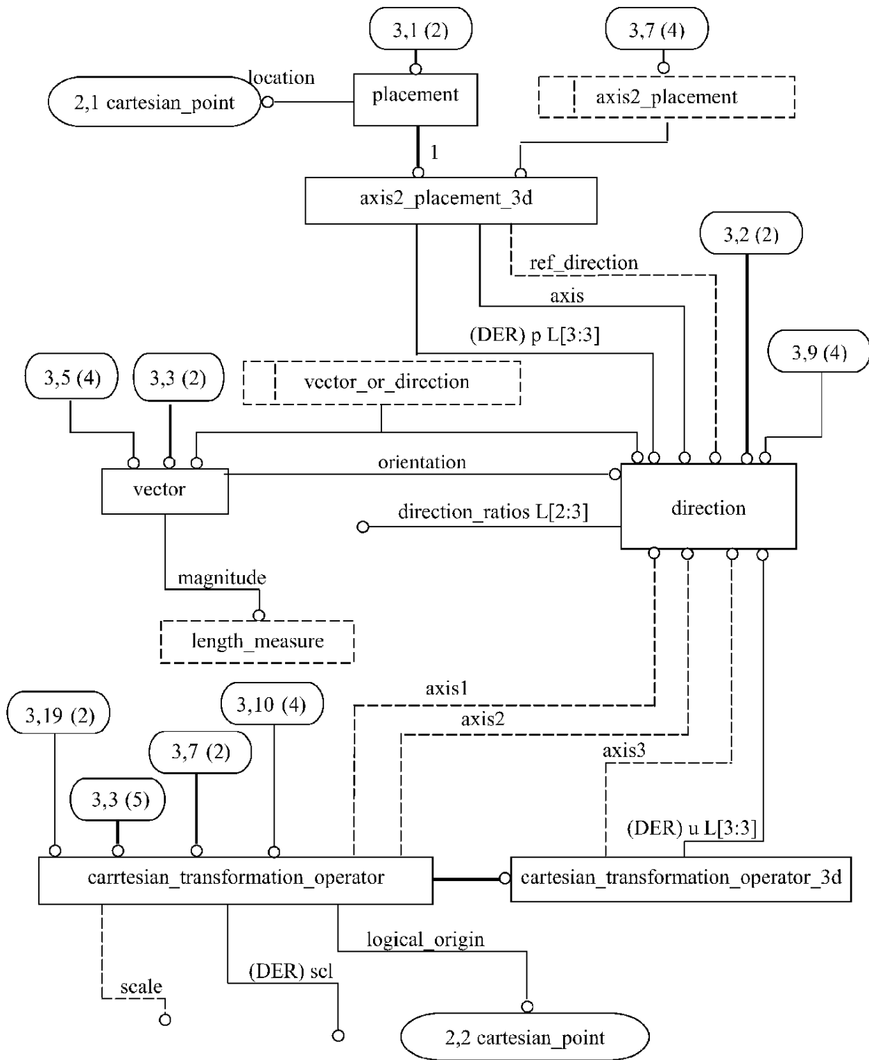
Рисунок С.3 — aic_edge_based_wireframe — EXPRESS-G диаграмма 3 из 6
