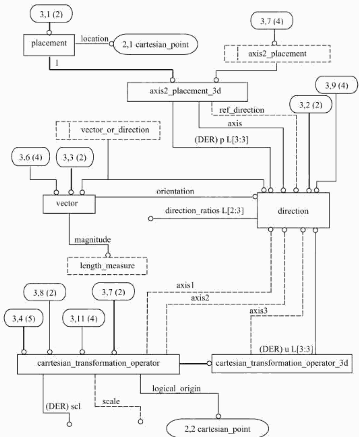
Рисунок С.3 — alc_shell_based_wireframe — EXPRESS-G диаграмма 3 из 6
