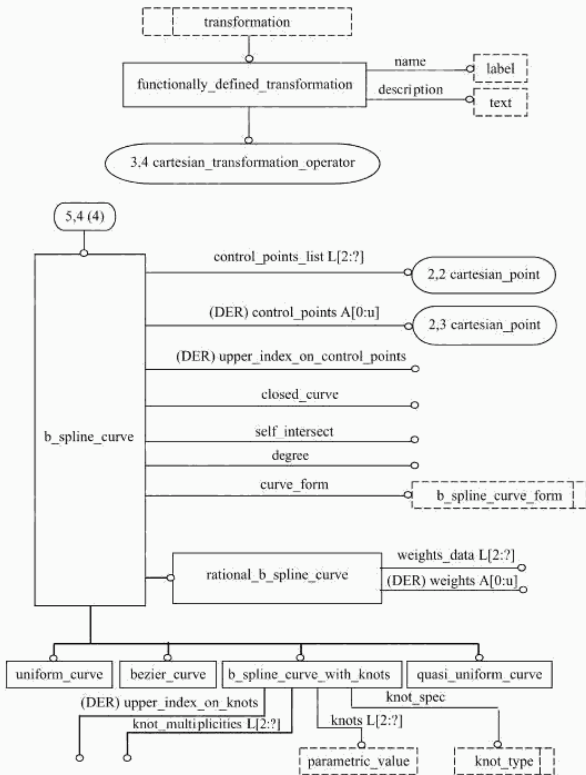
Рисунок С.5 — alc_shell_based_wireframe — EXPRESS-G диаграмма 5 из 6
