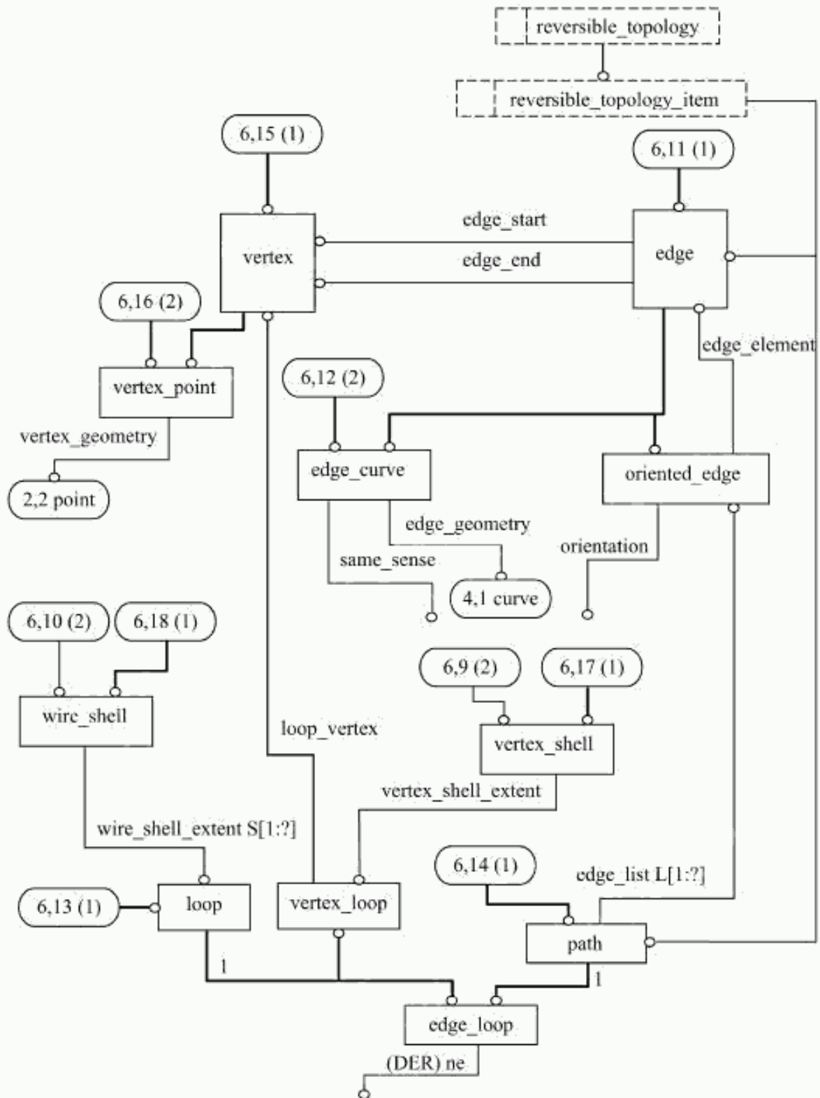
Рисунок С.6 — alic_shell_based_wireframe — EXPRESS-G диаграмма 6 из 6
