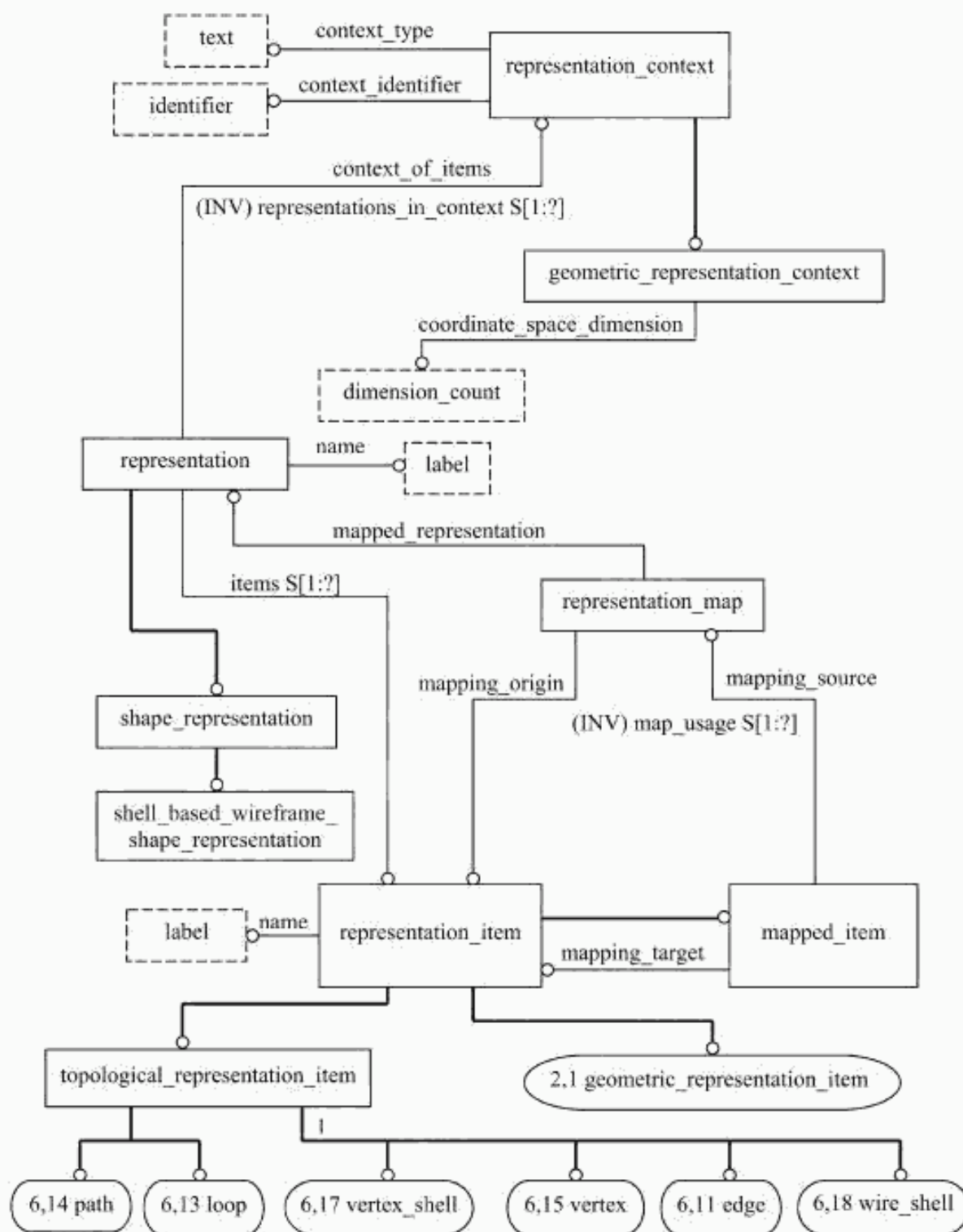
Рисунок С.1 — alc_shell_based_wireframe — EXPRESS-G диаграмма 1 из 6
