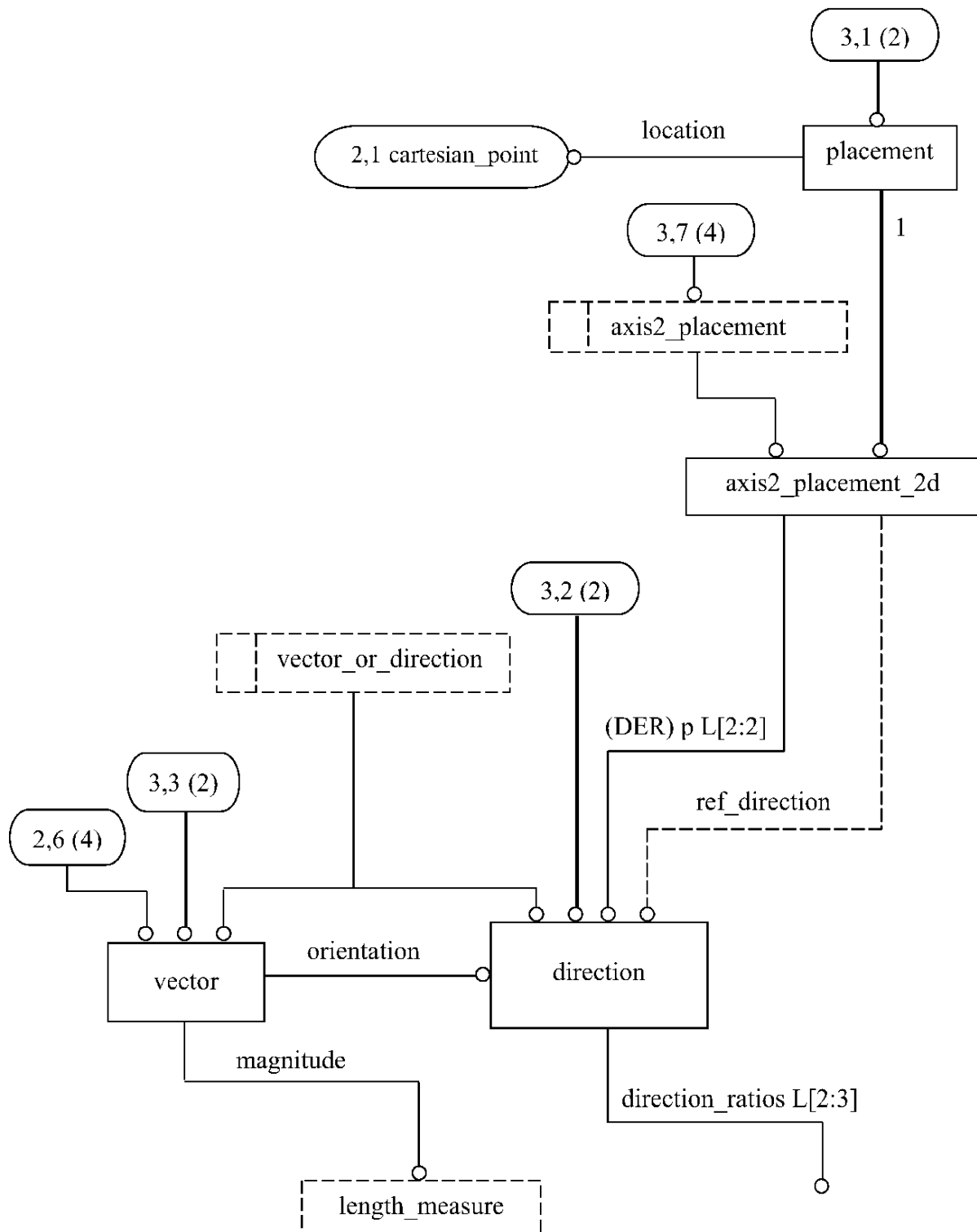
Рисунок С.3 — aic_geometrically_bounded_2d_wireframe — EXPRESS-G диаграмма 3 из 5
