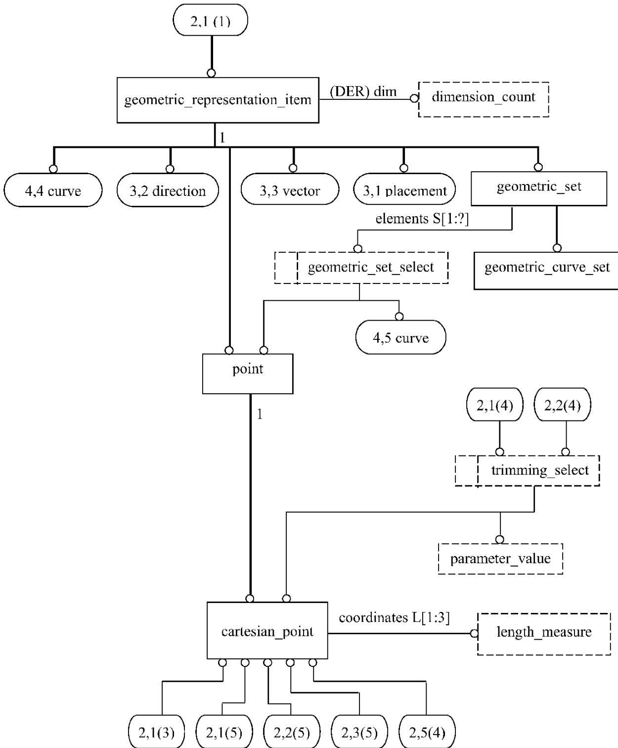
Рисунок С.2 — aic_geometrically_bounded_2d_wireframe — EXPRESS-G диаграмма 2 из 5
