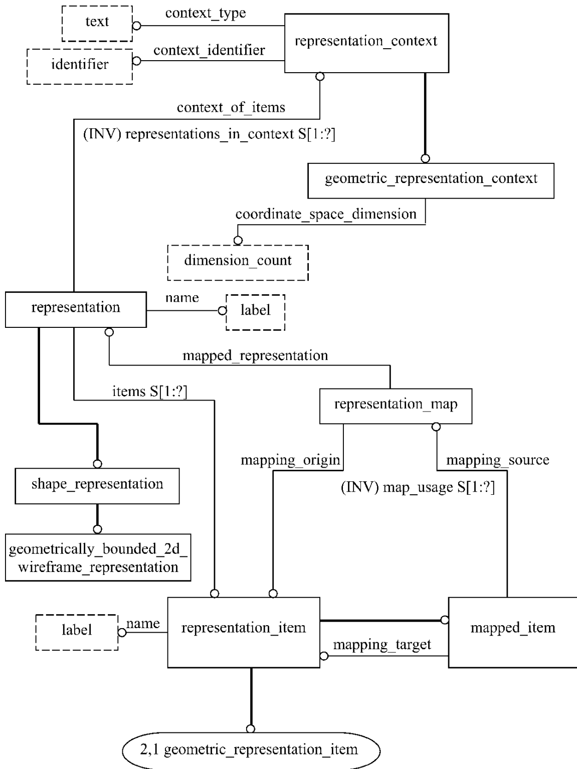
Рисунок С.1 — aic_geometrically_bounded_2d_wireframe — EXPRESS-G диаграмма 1 из 5
