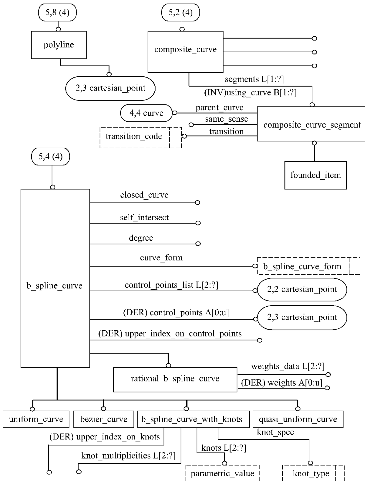
Рисунок С.5 — aic_geometrically_bounded_2d_wireframe — EXPRESS-G диаграмма 5 из 5
