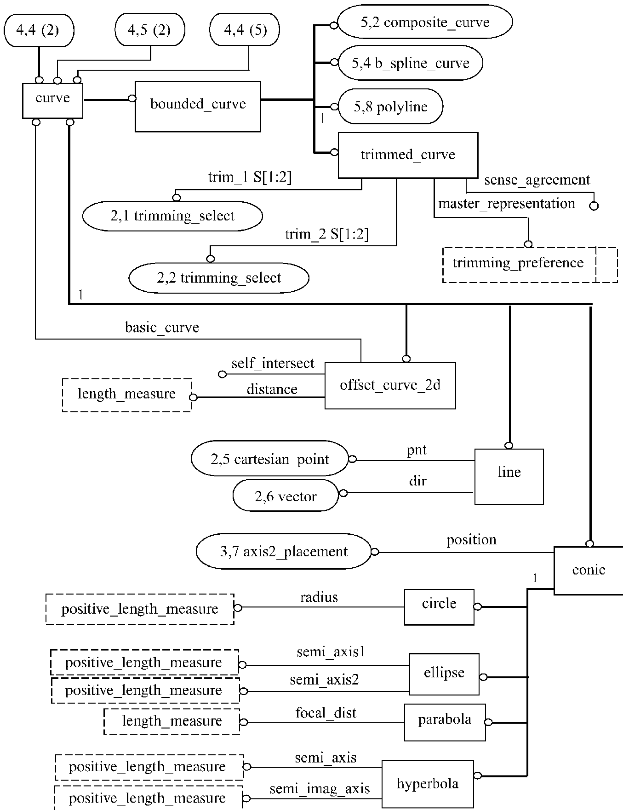
Рисунок С.4 — aic_geometrically_bounded_2d_wireframe — EXPRESS-G диаграмма 4 из 5
