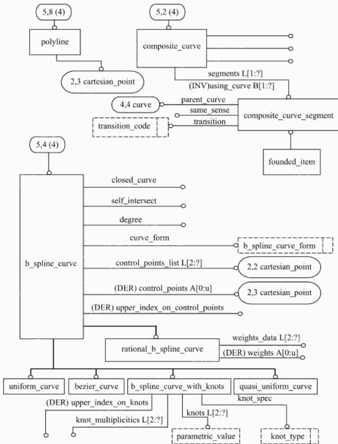
Рисунок С.5 — aic_geometrically_bounded_2d_wireframe — EXPRESS-G диаграмма 5 из 5
