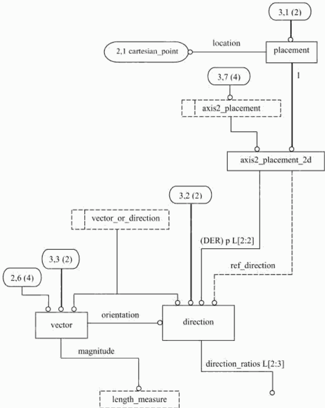
Рисунок С.3 — aic_geometrically_bounded_2d_wireframe — EXPRESS-G диаграмма 3 из 5
