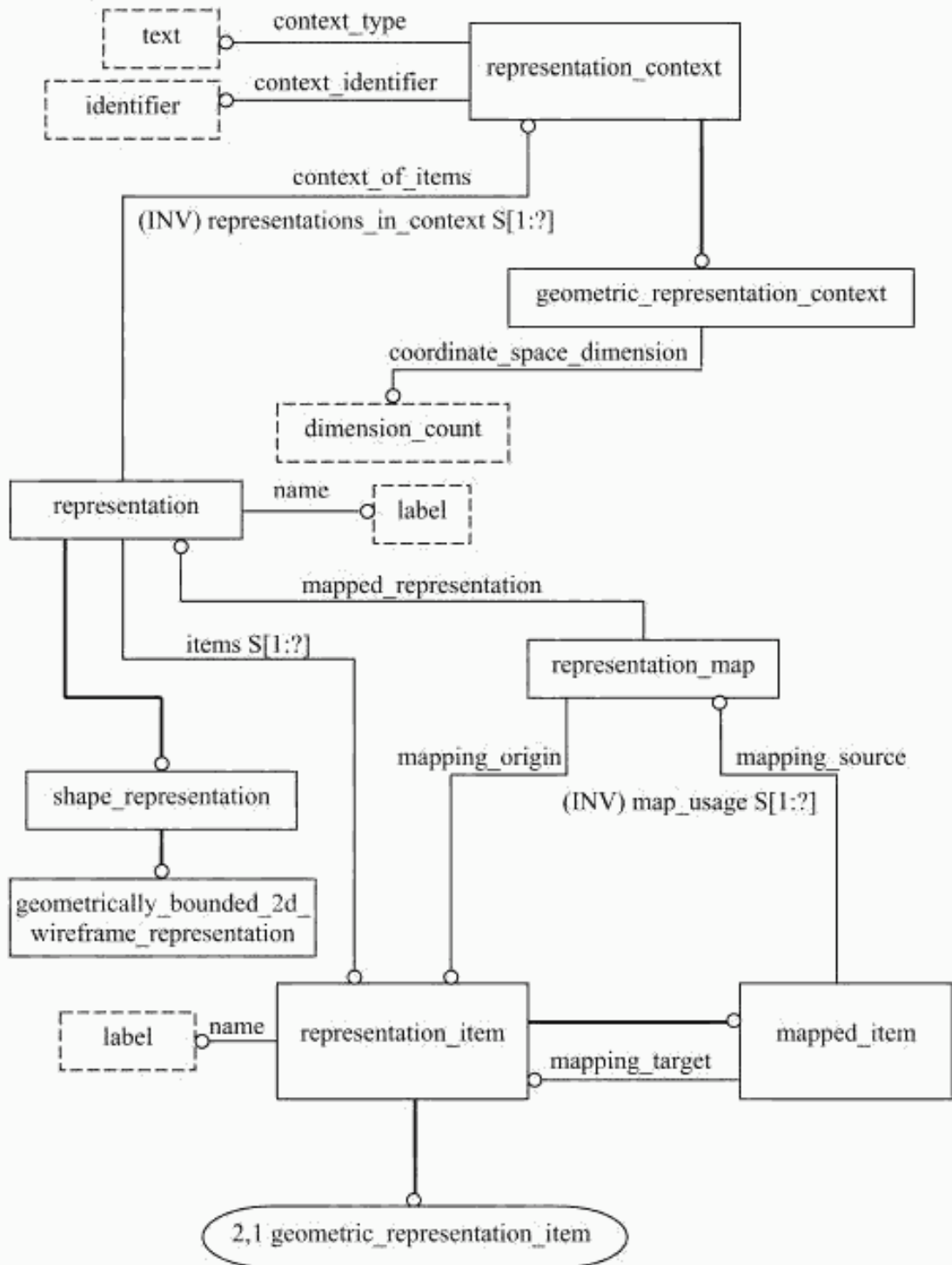
Рисунок С.1 — alic_geometrically_bounded_2d_wireframe — EXPRESS-G диаграмма 1 из 5
