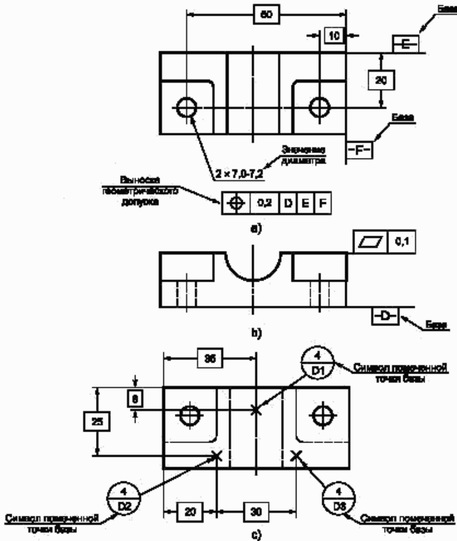
Рисунок 3 — Чертежные выноски
