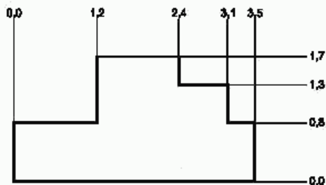
Рисунок 9 — Ординатный размер
