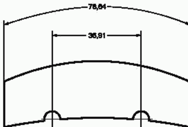
Рисунок 2 — Размер дуги
