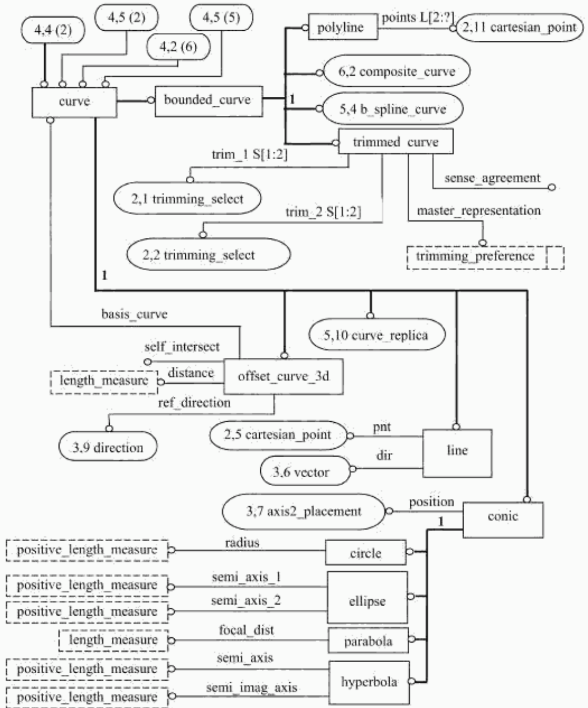
Рисунок С.4 — aic_geometrically_bounded_wireframe — EXPRESS-G диаграмма 4 из 6
