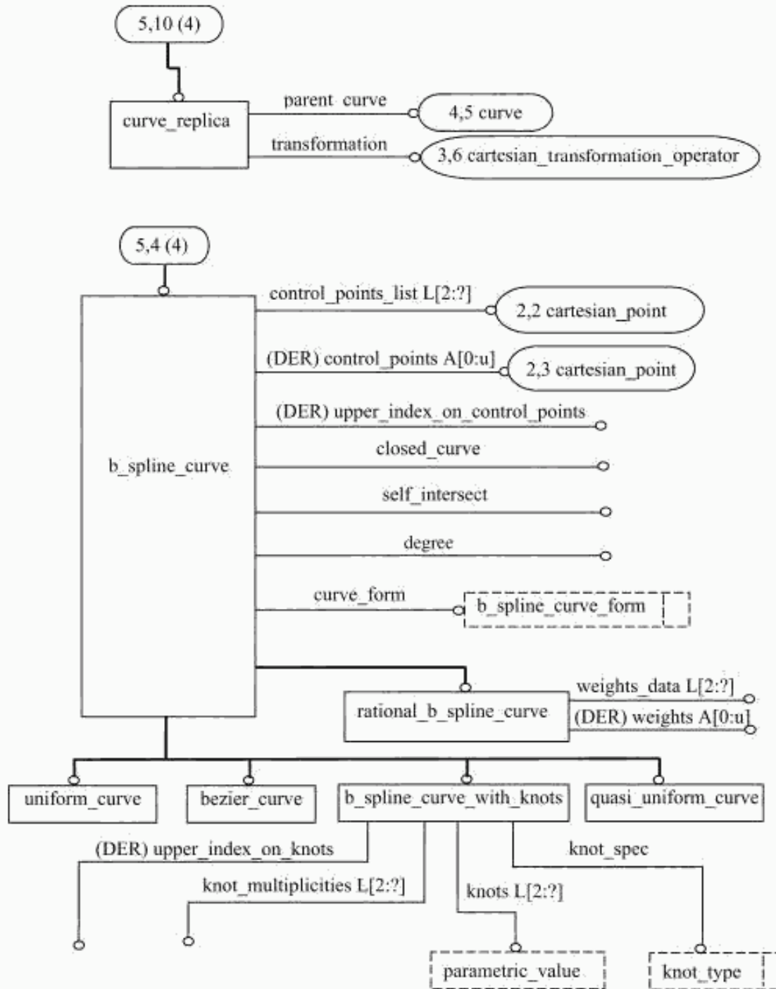
Рисунок С.5 — alc_geometrically_bounded_wireframe — EXPRESS-G диаграмма 5 из 6
