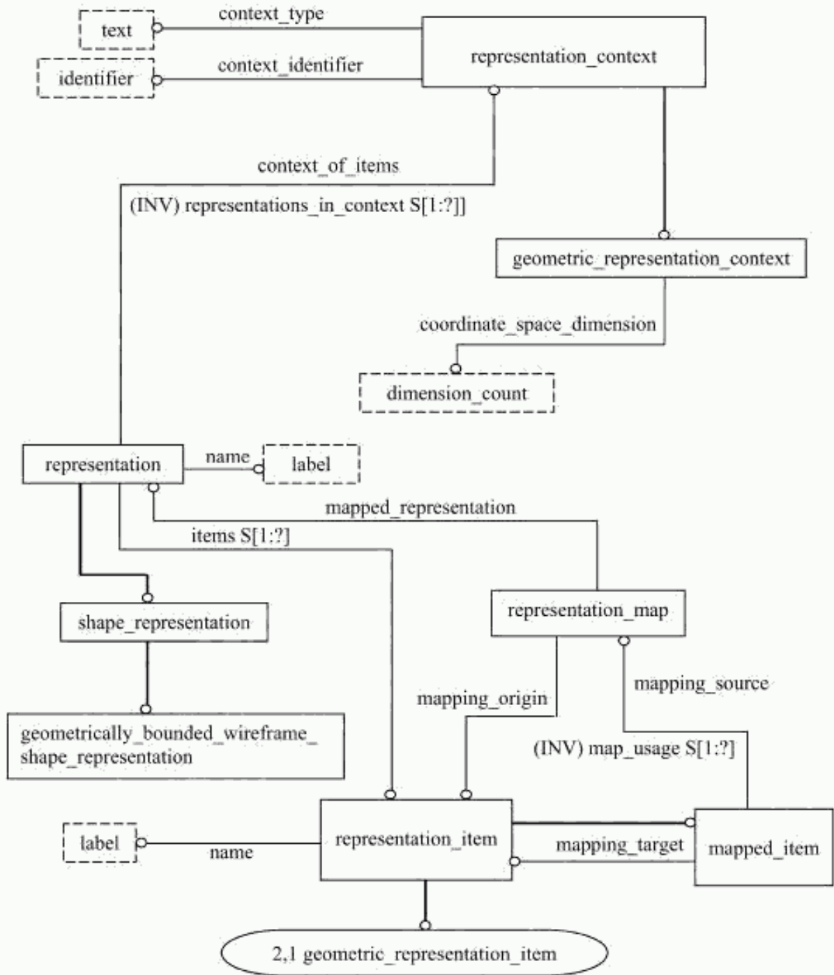
Рисунок С.1 — alic_geometrically_bounded_wireframe — EXPRESS-G диаграмма 1 из 6
