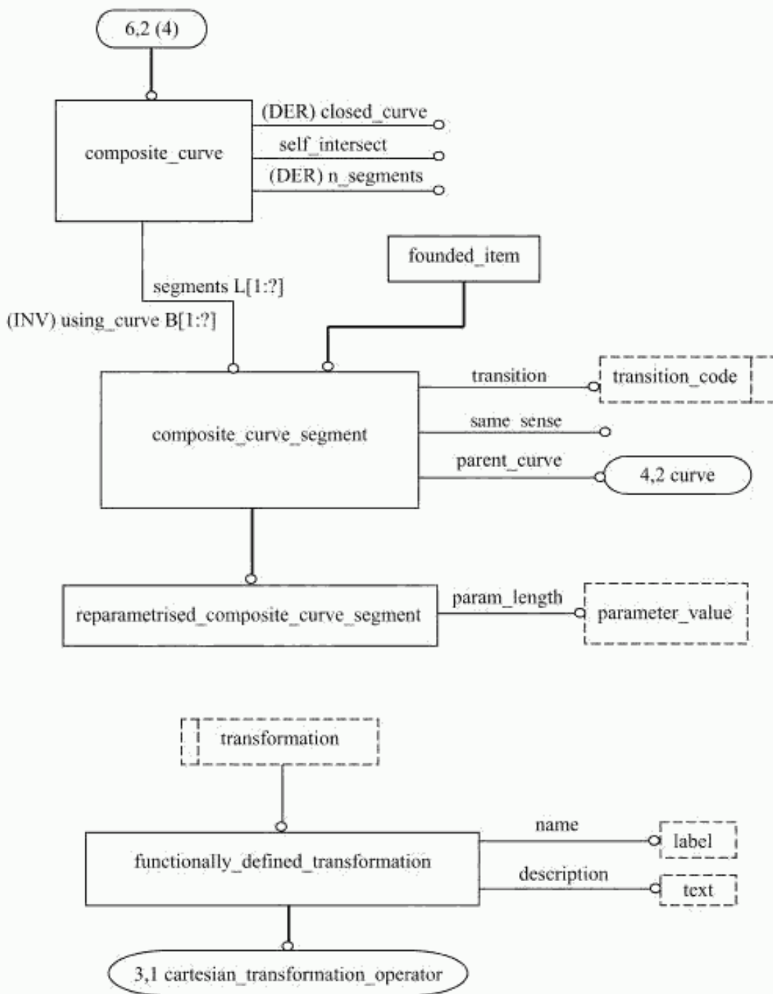
Рисунок С.6 — alic_geometrically_bounded_wireframe — EXPRESS-G диаграмма 6 из 6
