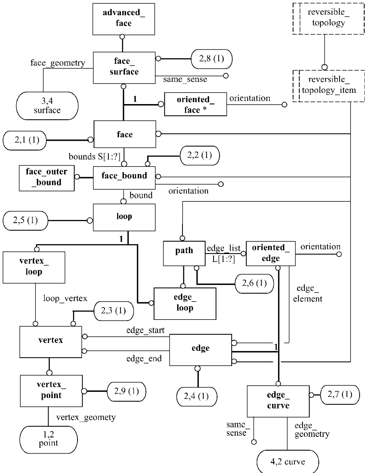
Рисунок D.2 — aic_topologically_bounded_surface — EXPRESS-G диаграмма 2 из 8
