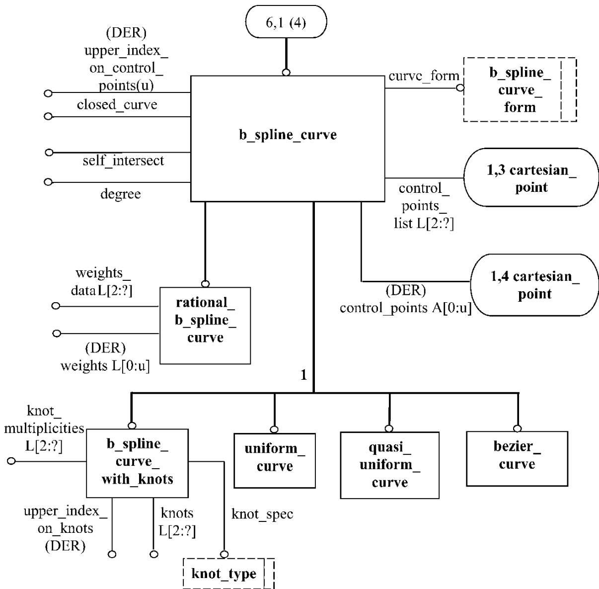
Рисунок D.6 — aic_topologically_bounded_surface — EXPRESS-G диаграмма 6 из 8
