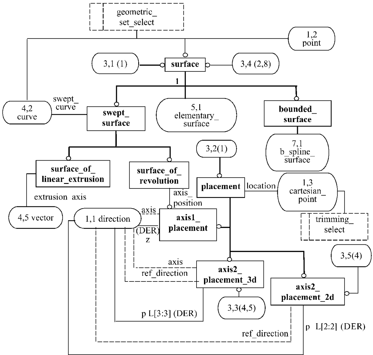
Рисунок D.3 — aic_topologically_bounded_surface — EXPRESS-G диаграмма 3 из 8
