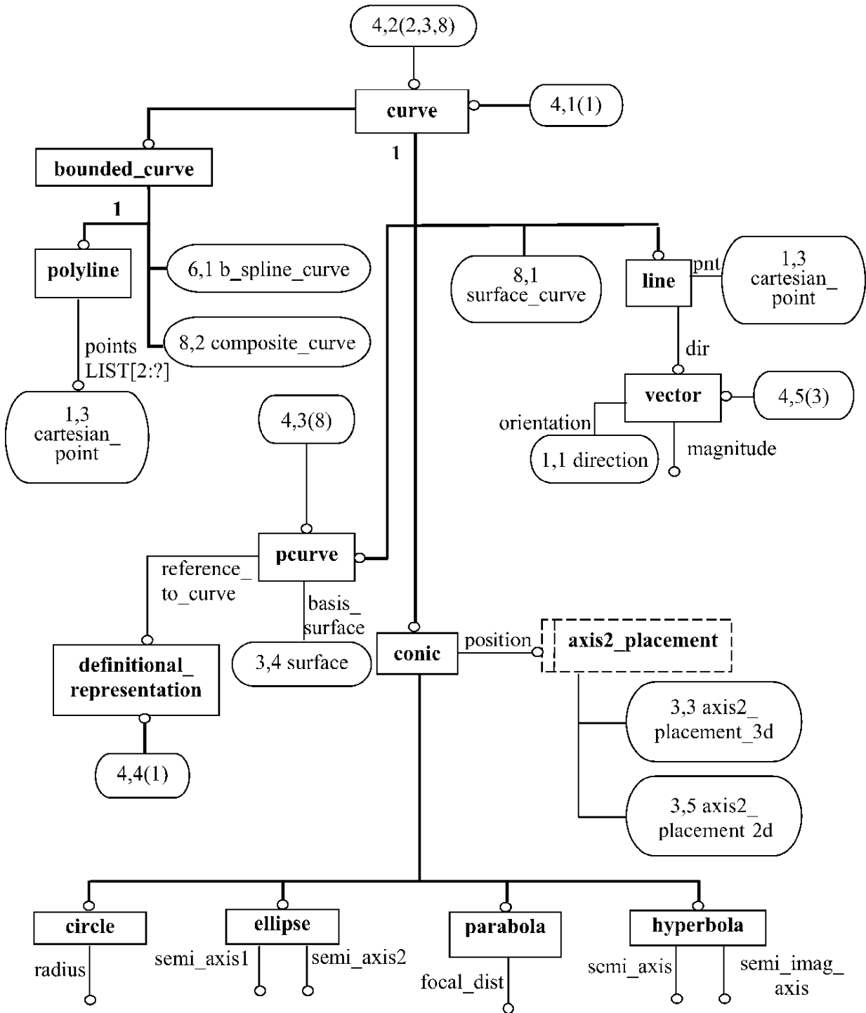
Рисунок D.4 — aic_topologically_bounded_surface — EXPRESS-G диаграмма 4 из 8
