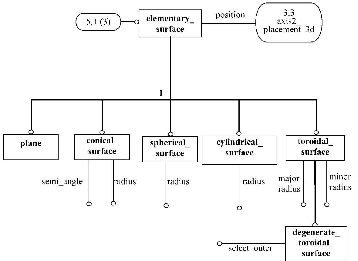
Рисунок D.5 — aic_topologically_bounded_surface — EXPRESS-G диаграмма 5 из 8
