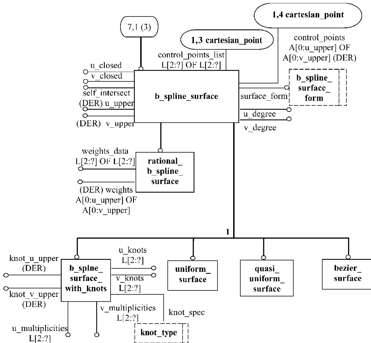
Рисунок D.7 — aic_topologically_bounded_surface — EXPRESS-G диаграмма 7 из 8
