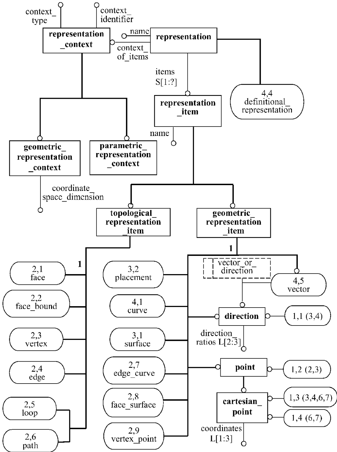
Рисунок D.1 — aic_topologically_bounded_surface — EXPRESS-G диаграмма 1 из 8
