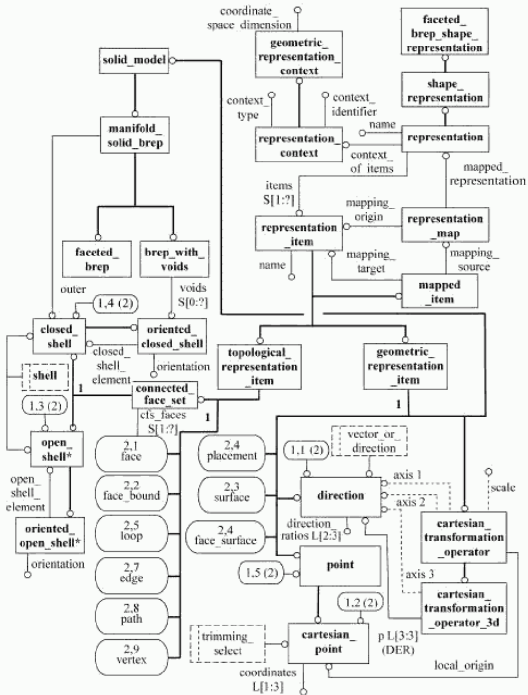
Рисунок D.1 — ПИК aic_faceted_brep в формате EXPRESS-G (диаграмма 1 из 2)
