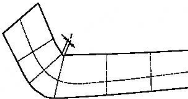
Рисунок 27 — Близкий к вырождению лоскут поверхности
