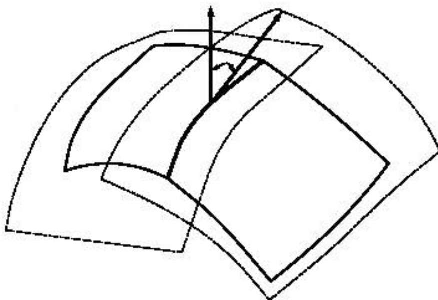
Рисунок 40 — Измерение разрыва G1 между гранями
