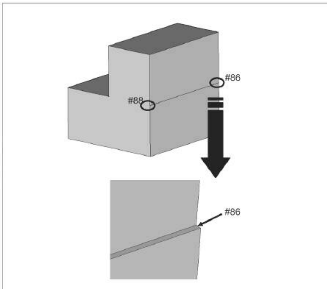
Рисунок Н.2 — Типичный пример ребра короткой длины
