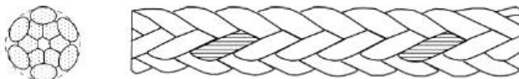
Рисунок 2 — Конфигурация 12-рядного плетеного каната (тип T)
