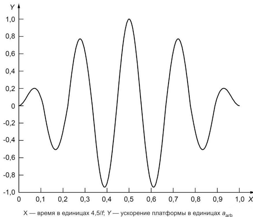
Рисунок А.1 — Сигнал ускорения платформы вибростенда
