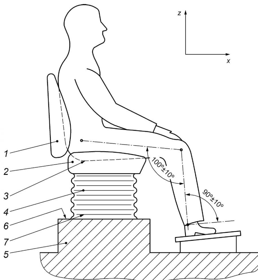
1 — спинка сиденья; 2 — подушка сиденья; 3 — установочный диск с акселерометром на подушке сиденья (S); 4 — подвеска сиденья; 5 — платформа вибростенда; 6 — акселерометр, установленный на поверхности платформы (P); 7 — опора сиденья
