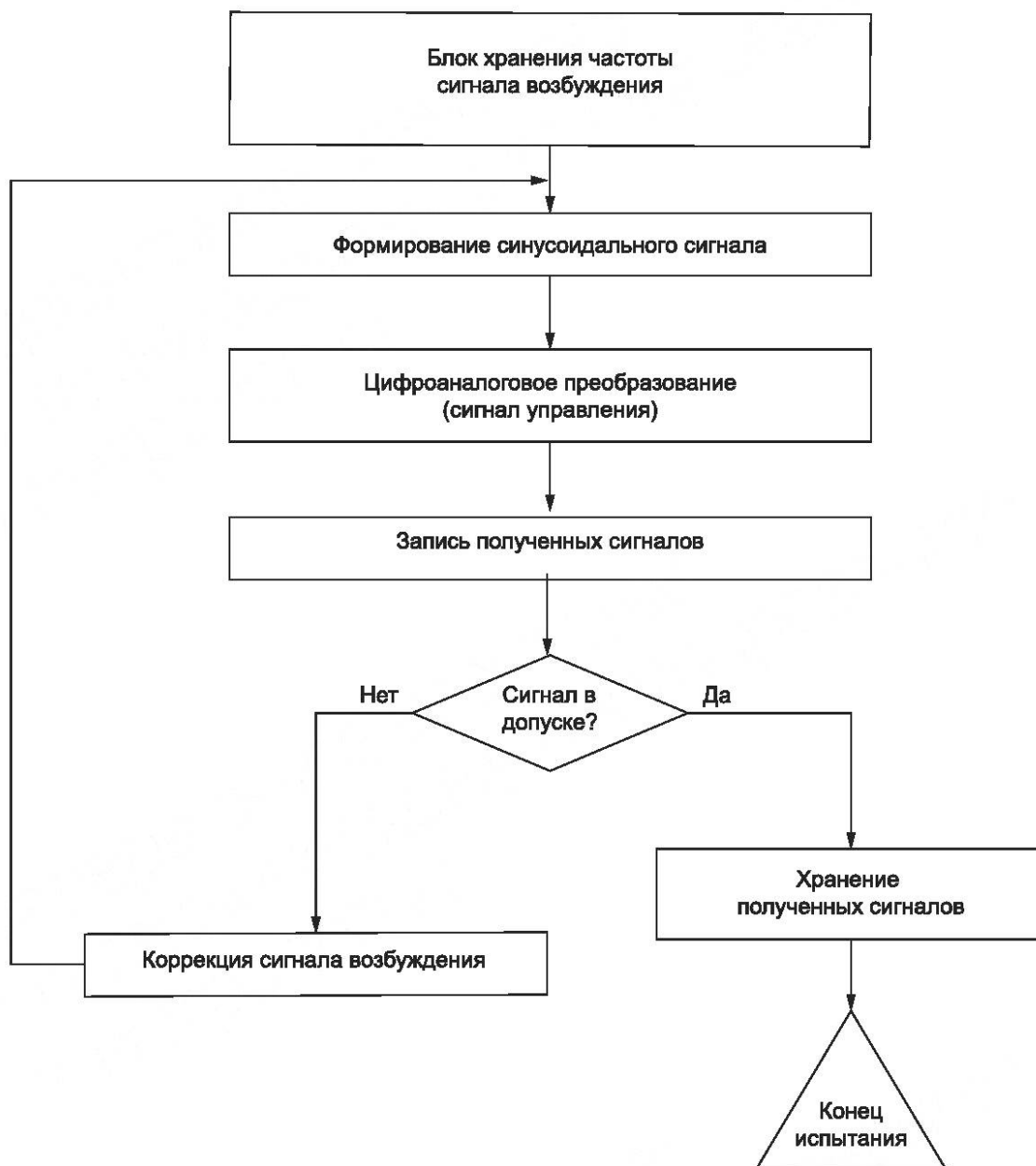
Рисунок A.2 — Блок-схема процедуры испытаний с возбуждением гармонической вибрации
