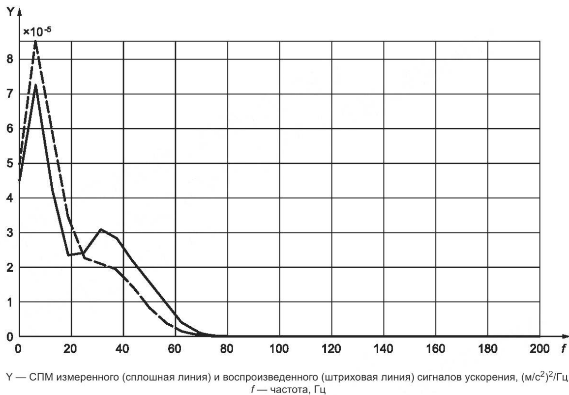
Рисунок В.4 — СПМ измеренного (вверху) и воспроизведенного (внизу) сигналов ускорения
