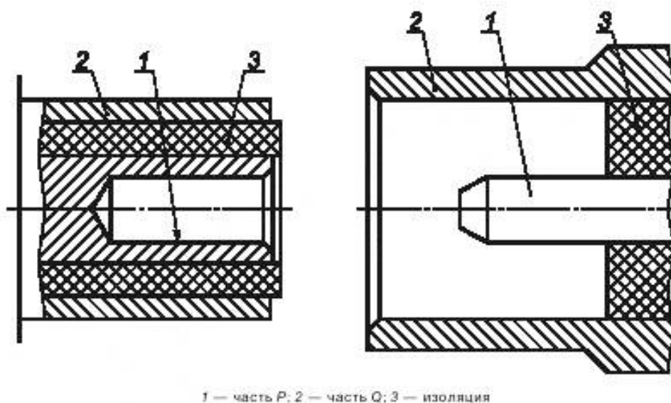
Рисунок 2 — Полярность гнезда и штекера соединителя миниатюрной фотовспышки портативных фотоаппаратов
