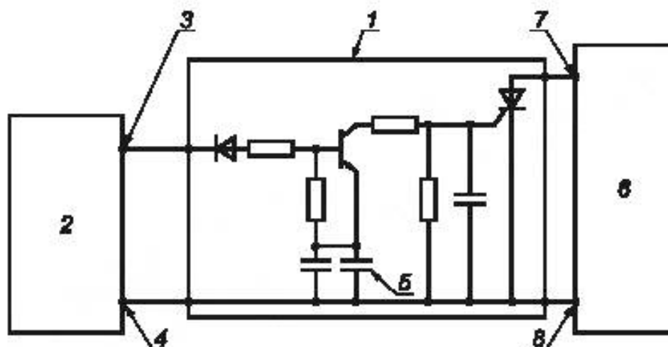
1 — адаптер; 2 — фотоаппарат; 3 — вывод синхронизатора с высоким потенциалом; 4 — вывод синхронизатора с низким потенциалом; 5 — батарея; 6 — блок фотовспышек; 7 — вывод цепи поджига с высоким потенциалом; 8 — вывод цепи поджига с низким потенциалом
