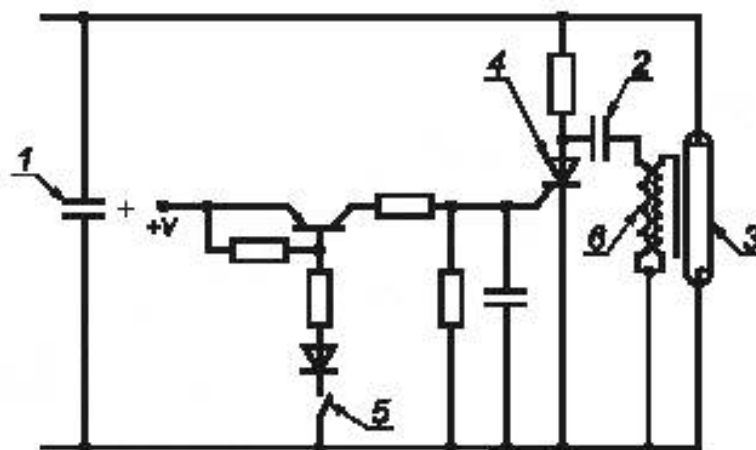
1 — основной конденсатор; 2 — триггерный конденсатор; 3 — ксеноновая газоразрядная трубка; 4 — резистор; 5 — выключатель синхронизатора; 6 — триггерный трансформатор
