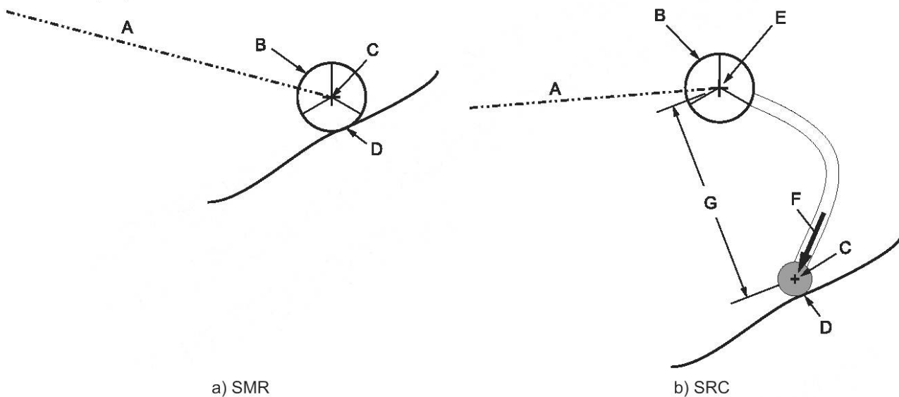
А — лазерный луч; В — светоотражатель (ретрорефлектор); С — точка измерения; D — точка контакта; Е — базовое местоположение; F — вектор нормали к перемещению щупа; G — смещение наконечника щупа
