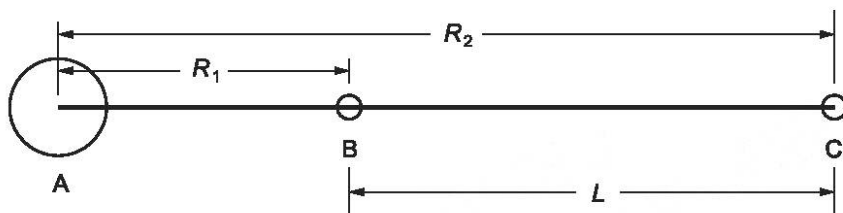
Рисунок D.2 — Конфигурация лазерного трекера для коллинеарных измерений
