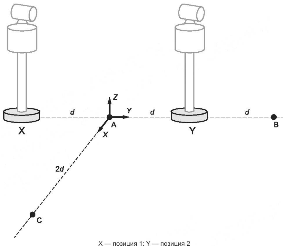
Рисунок Е.3 — Настройка для испытания инклинометра
