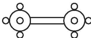
Рисунок С.1 — Вид, показывающий схему четырехточечного осязательного измерения сферы, используемый для двунаправленного измерения стержня со сферами
