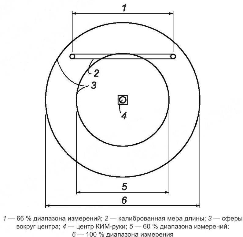
Рисунок 4 — Позиции для размещения калиброванной меры длины
