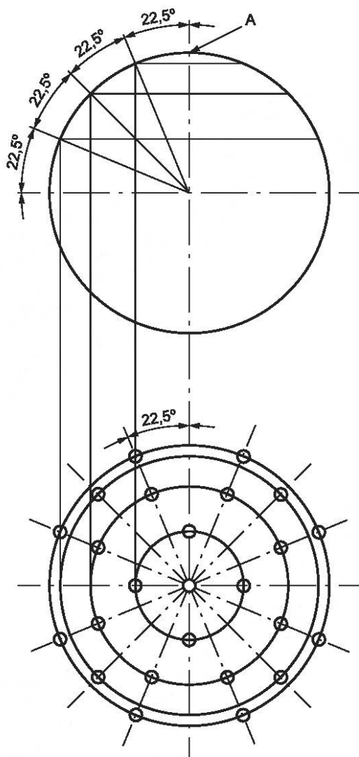
Рисунок 2 — Расположение точек ощупывания (А — полюс)
