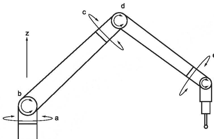
а) КИМ с шестью осями вращения
