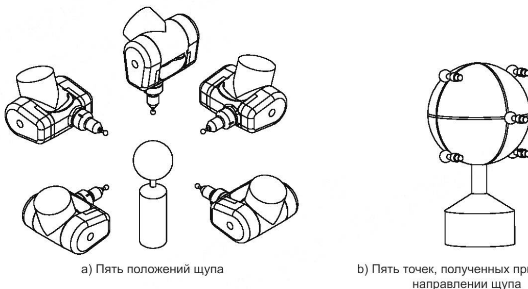
Рисунок 3 — Точки полюсов
