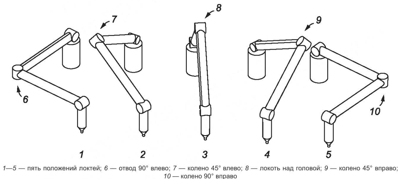
Рисунок D.1 — Вид, показывающий пять положений КИМ-руки при выполнении одноточечного испытания на артикуляцию
