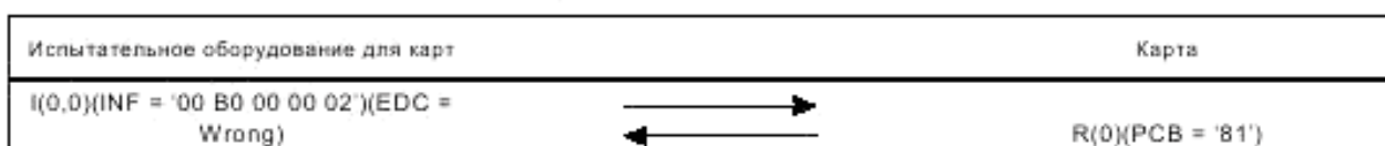
Сценарий 3 — Разграничительный интервал блока (BGT), методика 2
