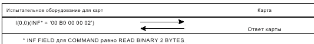
Сценарий 1 — Характер изменения времени ожидания знака (CWT)
