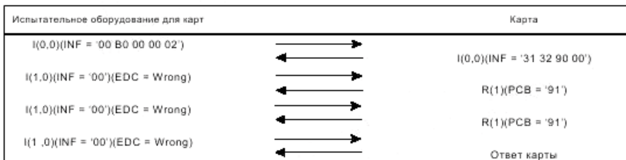
Сценарий 5 — Упорядочение блоков в карте, методика 2
