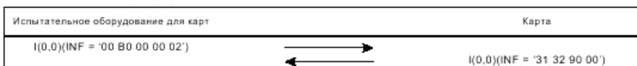
Сценарий 2 — Разграничительный интервал блока (BGT), методика 1
