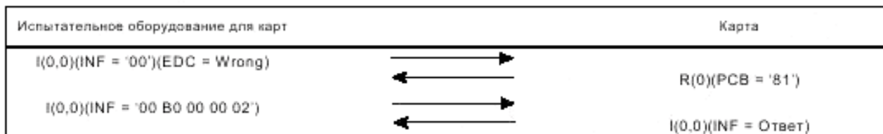
Сценарий 4 — Упорядочение блоков в карте, методика 1
