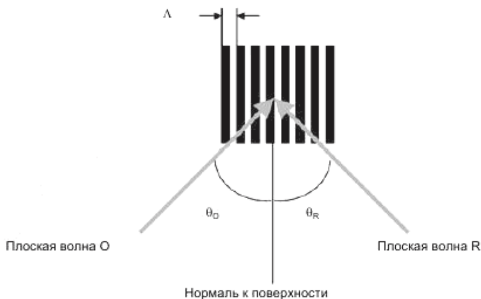
Рисунок 5 – Запись дифракционной решетки в запоминающем слое при помощи интерференции двух плоских волн
