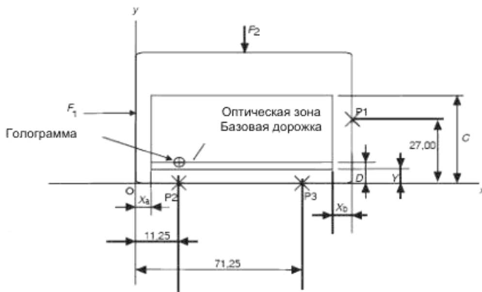
Рисунок 1 – Расположение оптической зоны и базовой дорожки
