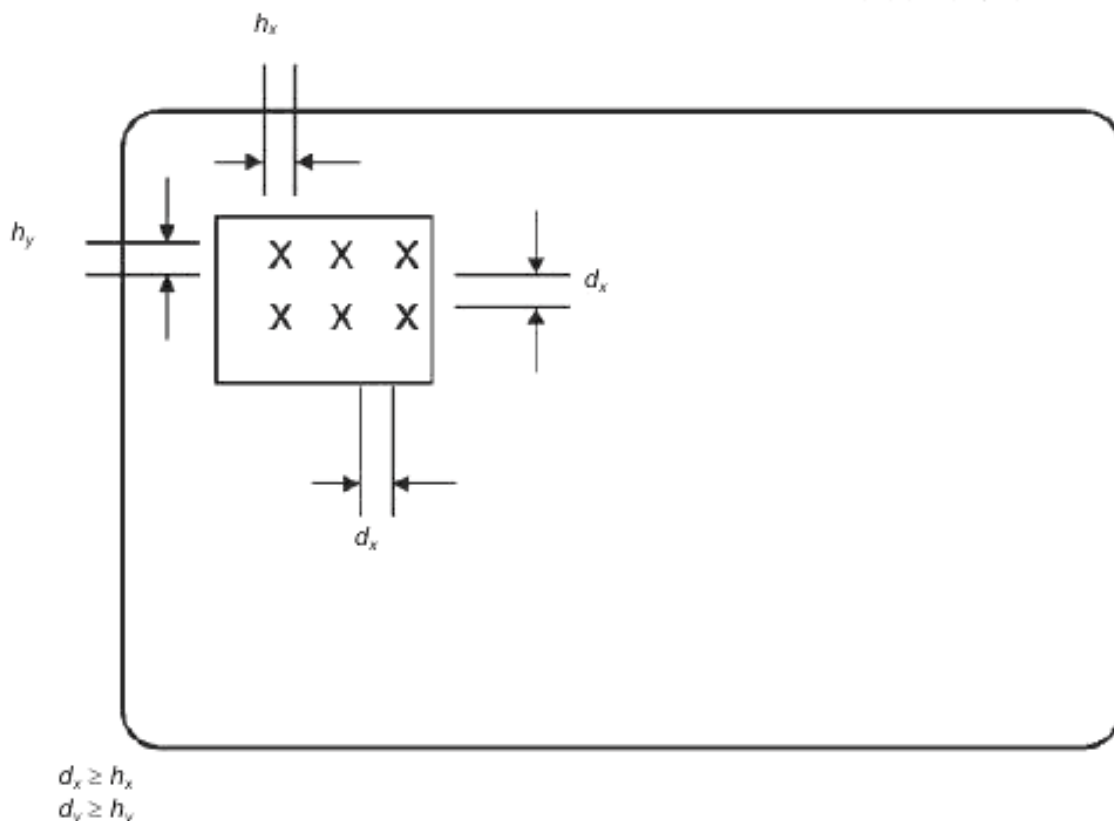
Рисунок 4 — Компоновка из нескольких голограмм
