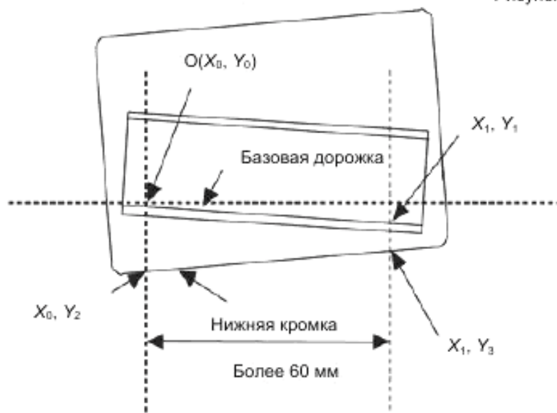
Рисунок 3 – Методика измерения наклона
