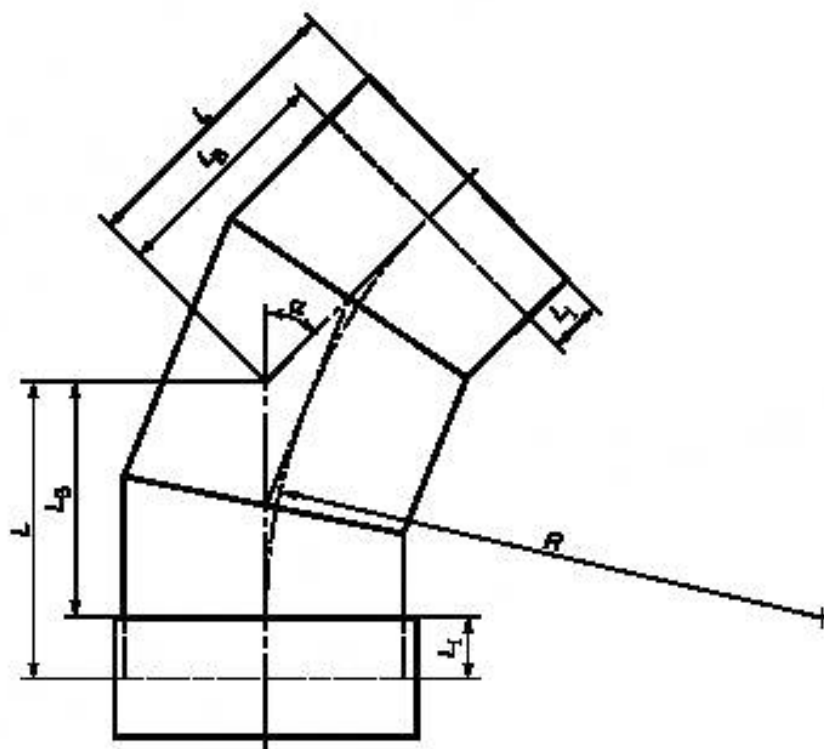
Рисунок 2 — Пример литого отвода
