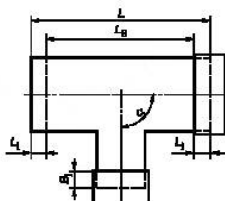
б — Неравнопроходной тройник
