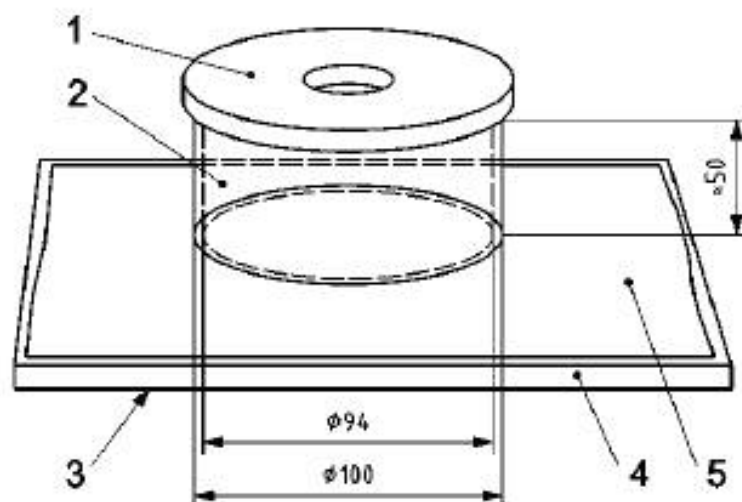
1 — нагрузочное кольцо; 2 — цилиндр; 3 — пластиковая пленка; 4 — полиуретановая подложка; 5 — образец для испытаний
