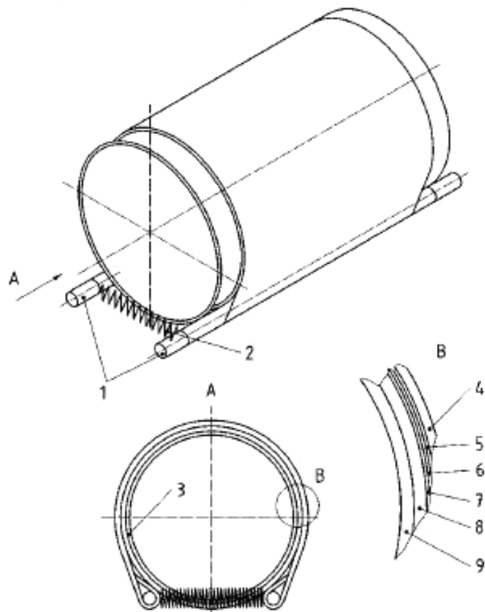
1 — стальные стержни; 2 — пружина для поддержания стальных стержней на месте с обеих сторон цилиндра; 3 — медный цилиндр (80 мм диаметр, 1,5 мм толщина); 4 — внешняя оболочка из хлопчатобумажной ткани; 5 — смежная ткань; 6 — образец для испытаний; 7 — смежная ткань; 8 — шесть слоев хлопчатобумажной ткани; 9 — медный цилиндр
