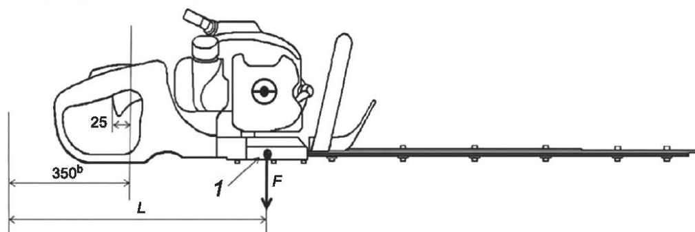
b) Расчет удерживающего момента на двустороннем кусторезе
