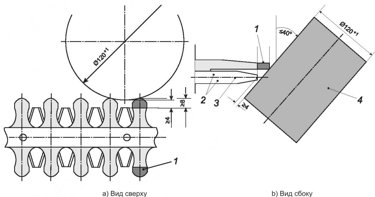
Рисунок 6 — Конфигурация режущего механизма
