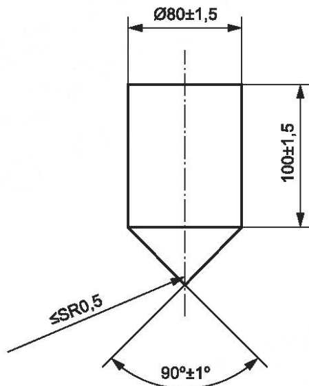
Рисунок 10 — Размеры конуса
