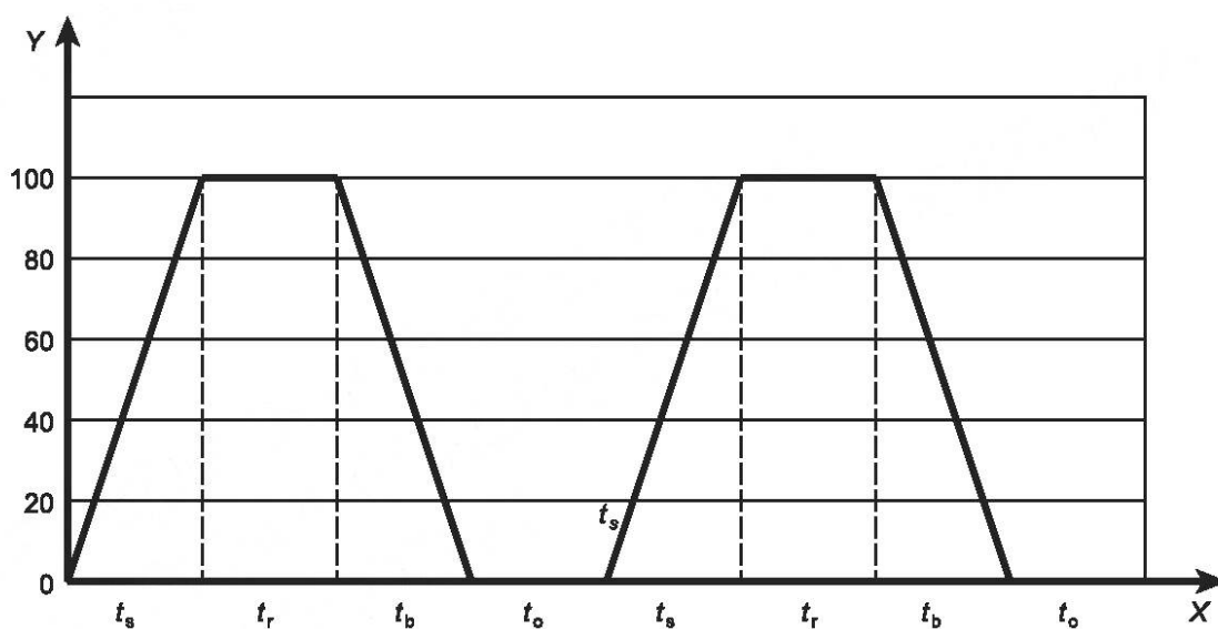
Рисунок 9 — Пример циклов испытаний
