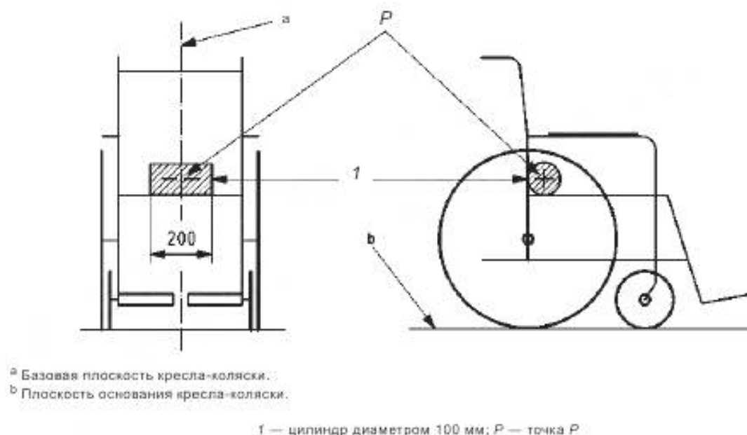
Рисунок 1 — Базовая точка P кресла-коляски и базовая плоскость кресла-коляски
