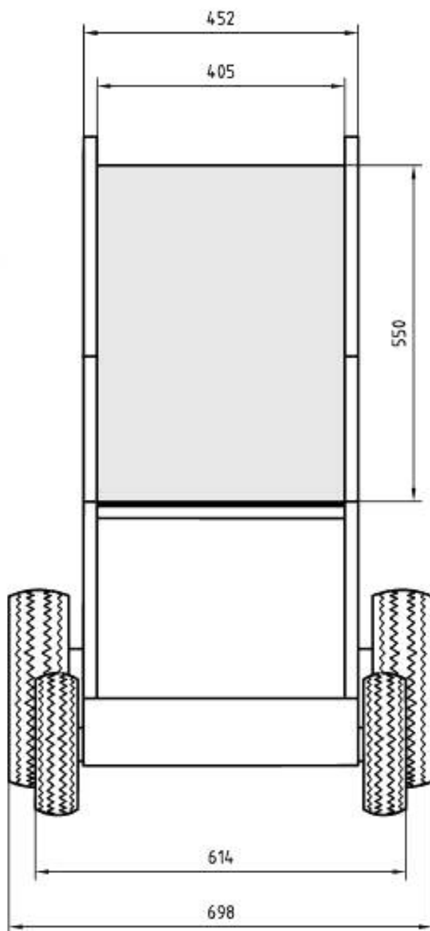
Рисунок Е.2 — Имитатор кресла-коляски, вид спереди
