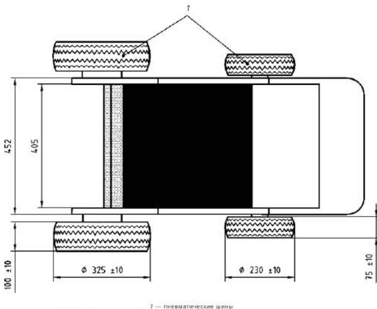
Рисунок Е.3 — Имитатор кресла-коляски, вид сверху
