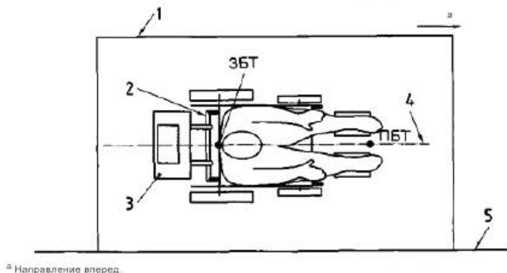
1 — наклоняющаяся испытательная платформа; 2 — адаптер соединения кресла-коляски; 3 — устройство стыковочного крепления; 4 — базовая плоскость кресла-коляски и средняя линия испытательной платформы; 5 — ось наклона испытательной платформы; ЗБТ — задняя базовая точка; ПБТ — передняя базовая точка.
