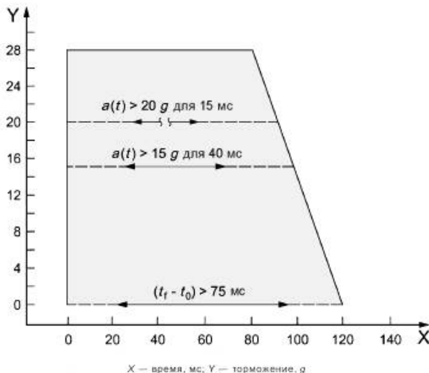
Рисунок А.1 — Требования по ускорению/торможению для испытания при лобовом столкновении при скорости (48 \pm 2) км/ч
