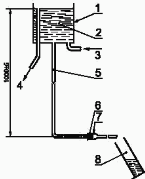
1 — резервуар постоянного уровня; 2 — дистиллированная или деионизированная вода; 3 — выпуск; 4 — слив; 5 — трубка для подачи воды; 6 — фитинг с 6 %-ным конусом Люэра с наружной резьбой; 7 — испытуемый катетер; 8 — сосуд для сбора/измерения
