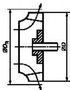
Рисунок 1 — Рабочее колесо радиального вентилятора
