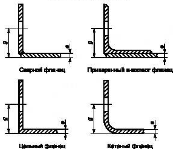
б) Различные варианты крепления
