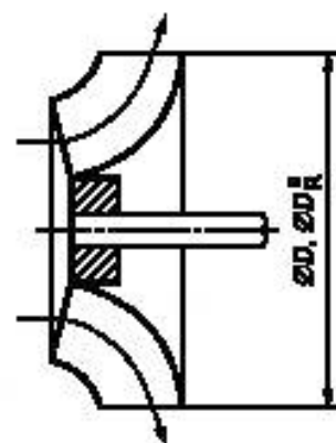
Рисунок 3 — Рабочее колесо диагонального вентилятора
