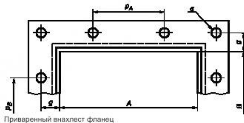
а) Расположение отверстий
