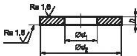
Рисунок 1 — Шайба типа N
