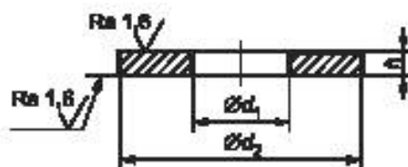
Рисунок 2 — Шайба типа L
