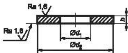
Рисунок 1 — Шайба типа S
