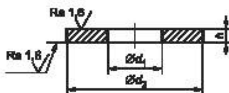
Рисунок 2 — Шайба типа N
