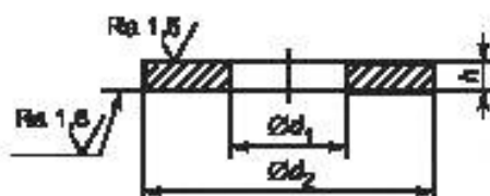
Рисунок 3 — Шайба типа L
