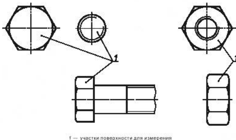
Рисунок 3 — Участки поверхности для измерения местной толщины слоя на крепежных изделиях
