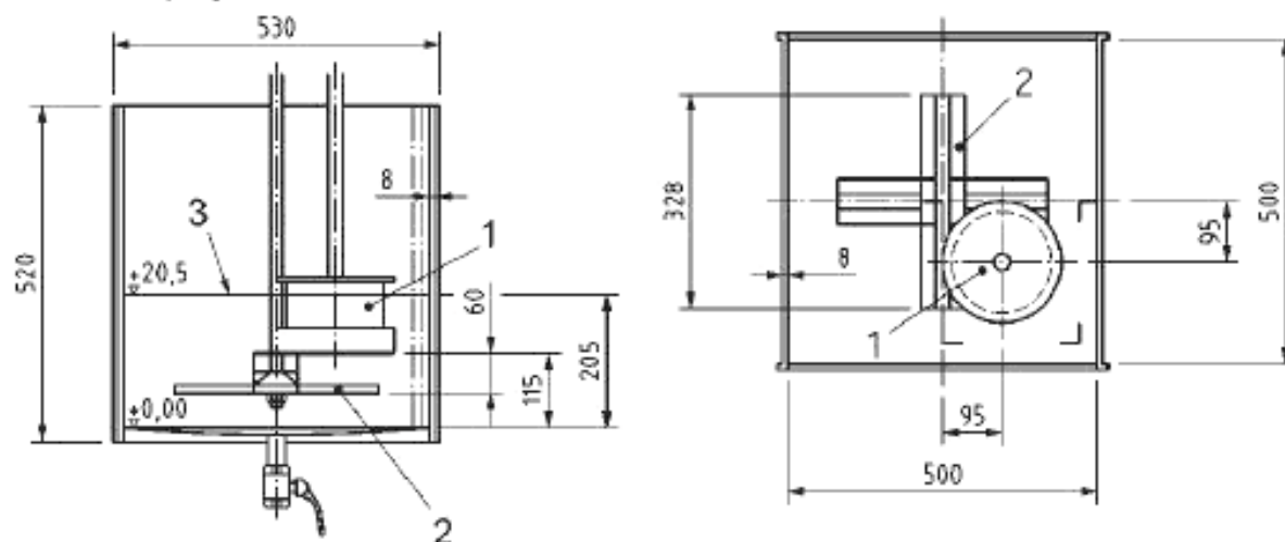
а) Чертеж отдельного испытательного контейнера – Вид сбоку и сверху в разрезе
