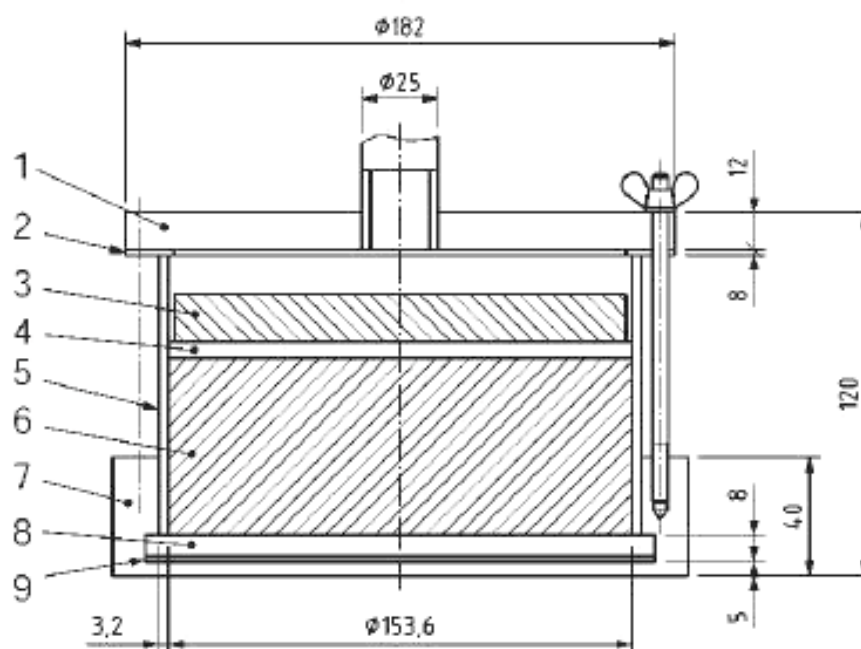
а) Чертеж отдельного испытательного контейнера – Вид сбоку и сверху в разрезе
