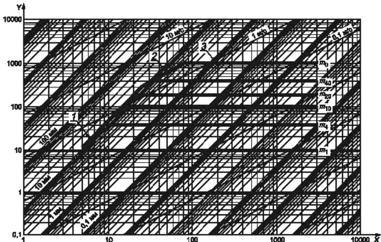
Рисунок 2 — Типичные характеристики электродинамического вибростенда
