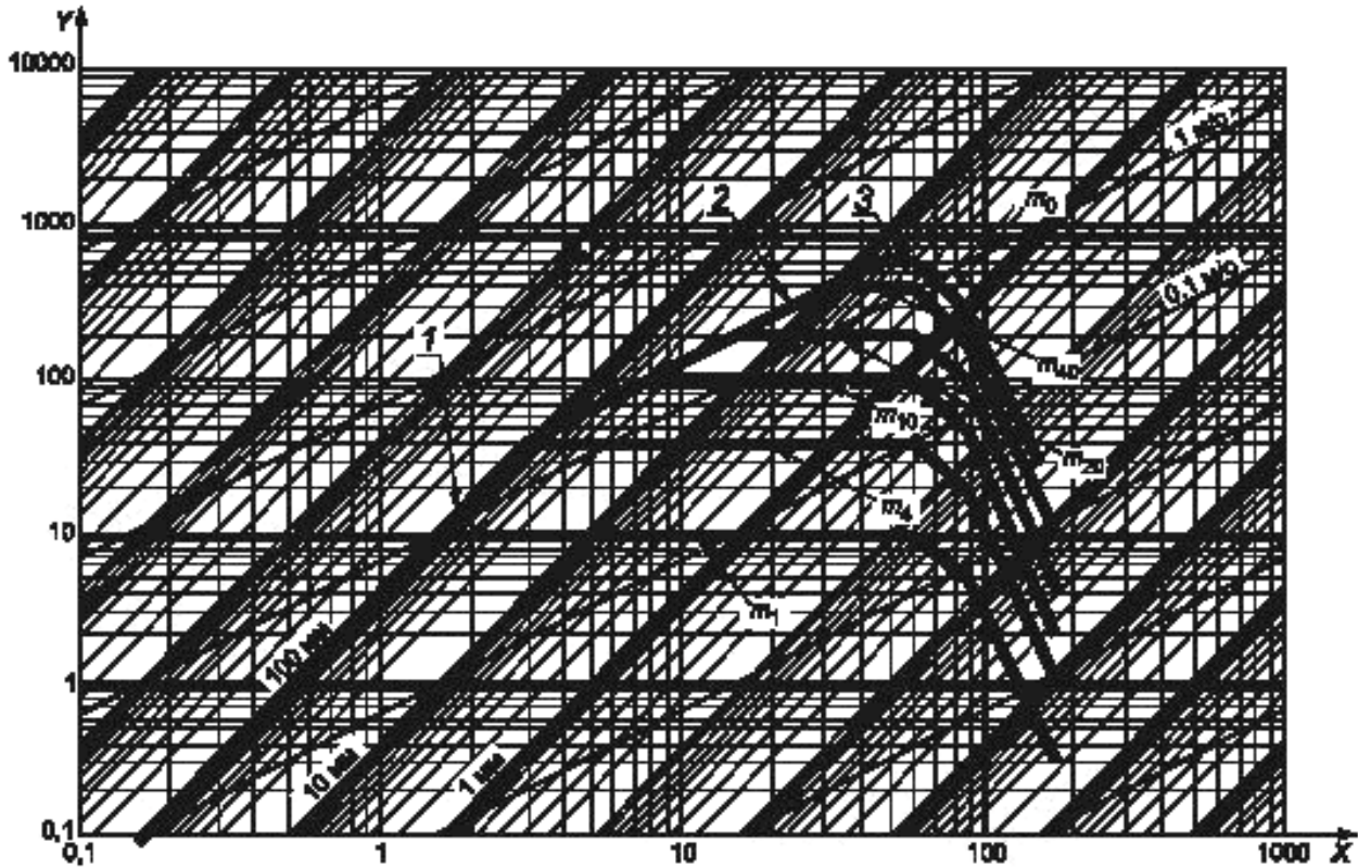
Рисунок 4 — Типичные характеристики гидравлического вибростенда
