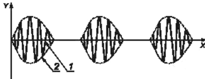
Рисунок 1 — Типичная последовательность синусоидальных импульсов с заполнением
