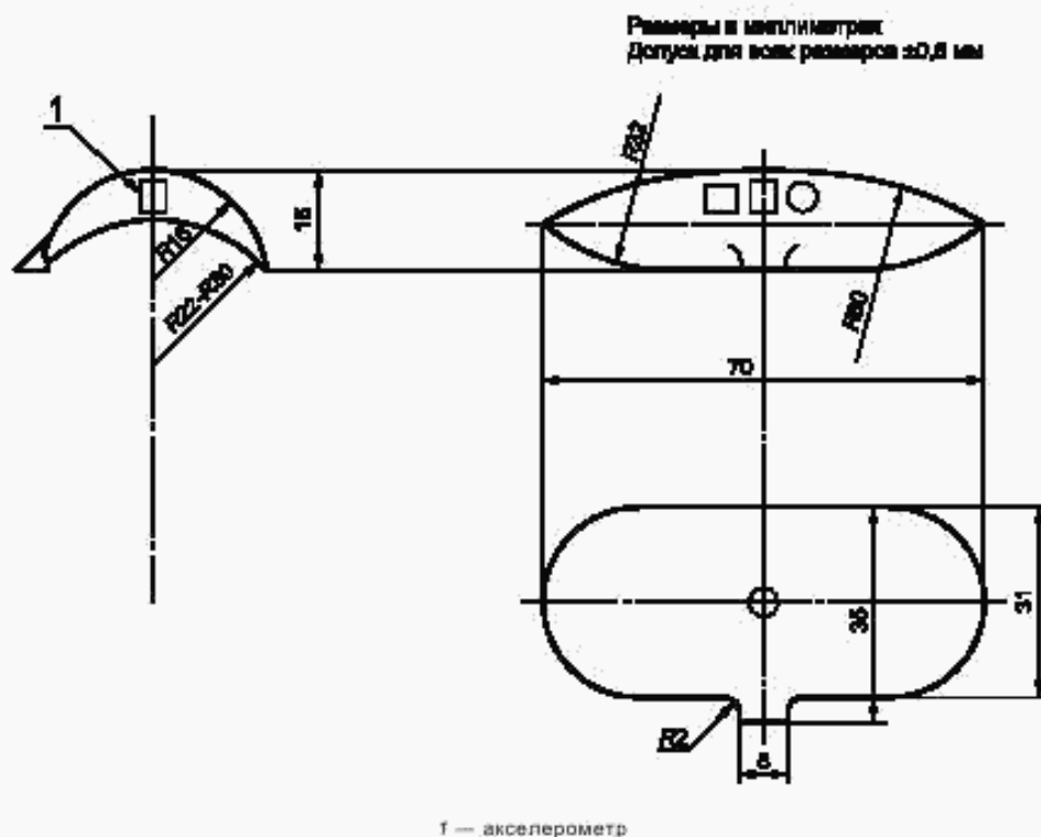
Рисунок 2 — Адаптер, позволяющий удерживать акселерометр в ладони руки
