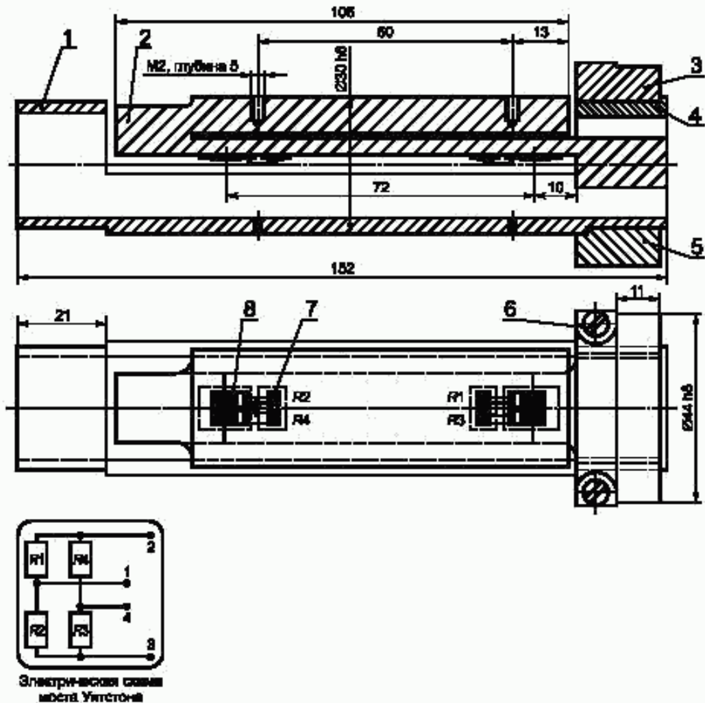
1 — рукоятка; 2 — измерительная пластина; 3 — стягивающее кольцо; 4 — площадка крепления; 5 — стягивающее кольцо; 6 — болт M2 × 16; 7 — паяный контакт; 8 — тензодатчик
