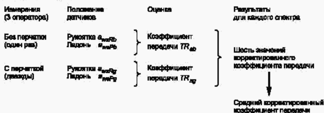
Рисунок 7 — Схема определения среднего скорректированного коэффициента передачи
